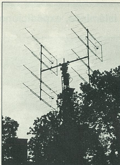
Ocho antenas de 11 elementos del conocido «moonbouncer» OK2PZW. (Foto cortesía de EA3ADW).
