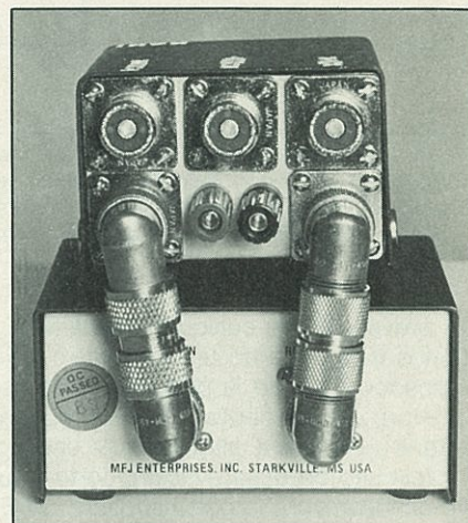
Vista posterior de las dos unidades. Obsérvese la utilización de conectores y adaptadores coaxiales para lograr una unión rígida de ambas unidades.
