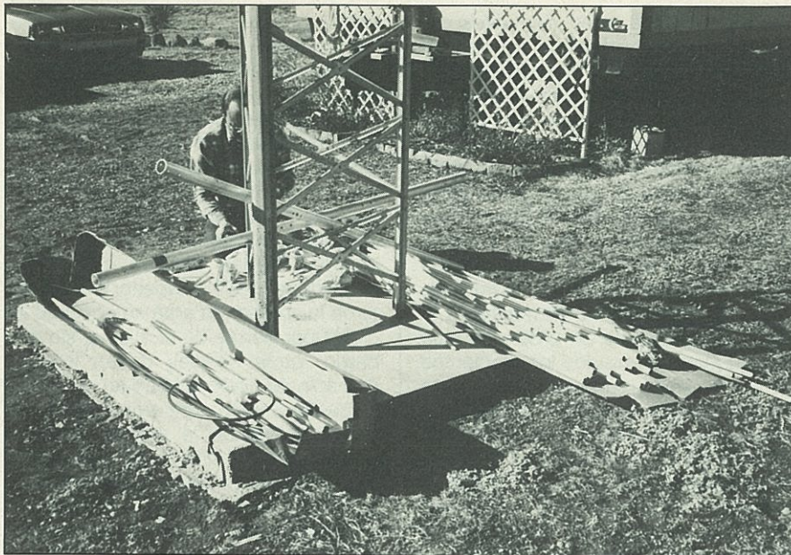
¡Todo listo para iniciar el montaje! La antena viene de fábrica en dos cajas de cartón.
