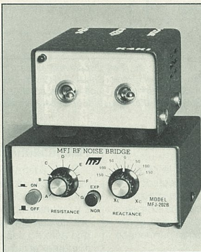
Vista frontal de la combinación de la unidad conmutadora y el puente de ruido MFJ.
