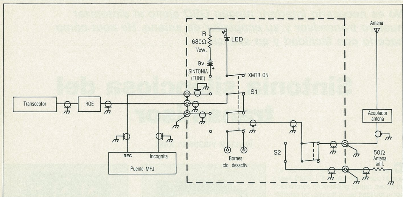
Figura 1. Esquema de la unidad conmutadora. El rectángulo de línea discontinua indica los límites de la cajita metálica en cuyo interior se monta la unidad. En el caso aquí descrito se utilizó una cajita Radio Shack 270-251A. Los componentes incluyen un conector de pila, los conectores coaxiales para chasis, dos bornes de nilón y la tornillería. Todo ello se puede adquirir fácilmente en cualquier tienda del ramo. El LED con intermitente incorporado fue el Radio Shack 276-036. Véase el texto para los detalles de los demás componentes del montaje.
