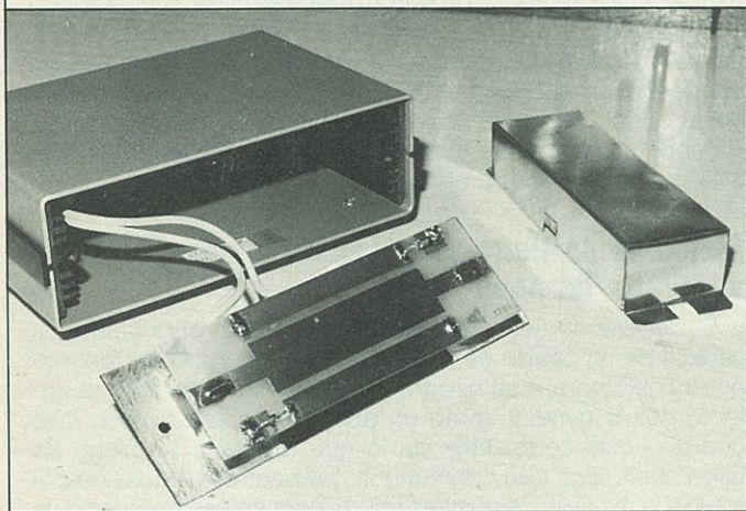
Figura 5. A la derecha, el blindaje que cubrirá el circuito del medidor que ya tenemos a punto de instalar en su caja metálica.
