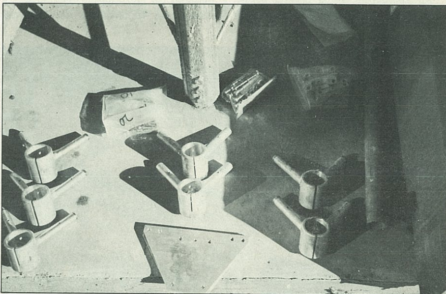
Las piezas en forma de V están destinadas a sujetar los elementos al travesaño. La pieza triangular es una de las unidades que sujetan el travesaño al mástil.
