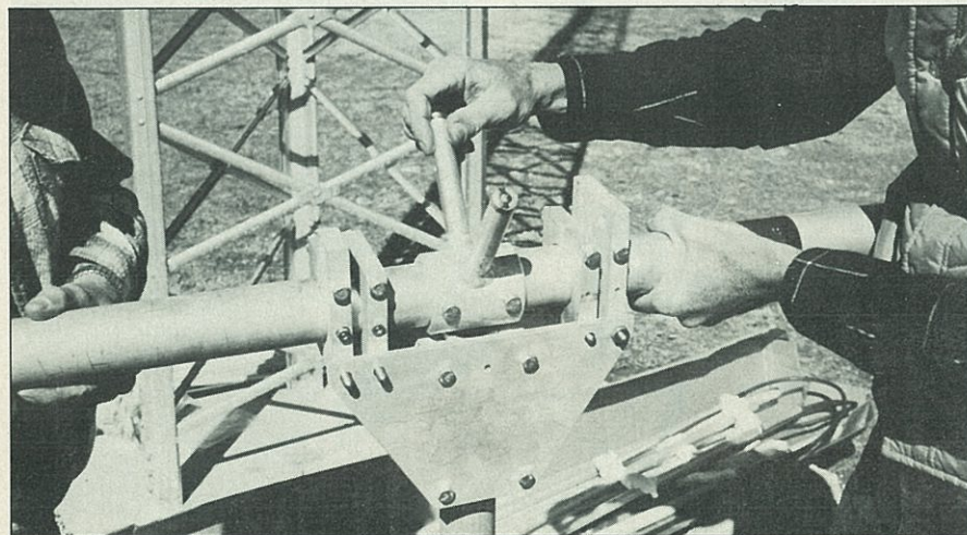
Podemos ver el soporte del travesaño en el mástil. Quitando tres tornillos, el travesaño puede pivotar sobre el cuarto tornillo. Lo probamos en la torreta y la cosa resultó FB.
