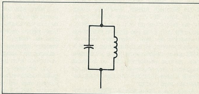
Figura 1. Esquema de una trampa de onda de antena.
