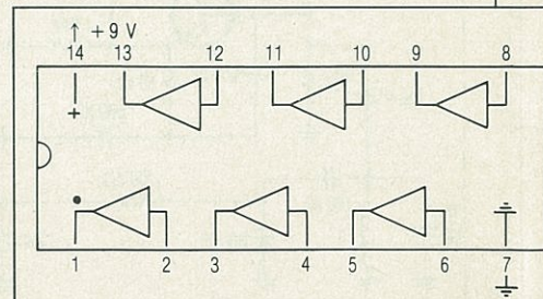
Figura 5. Disposición de las patillas del circuito integrado CD4069 de Philips, Toshiba, etc. Visto por encima.
