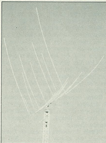
La antena delta tribanda montada en la cúspide de la torreta de 15 m de altura. Como se indica en el texto, las secciones radiantes superiores quedan a considerable mayor altura; a 21 m sobre el suelo en la banda de 20 metros, por ejemplo.
