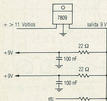
Figura 3. Alimentación positiva de los diferentes circuitos. Todos se desacoplan individualmente con una resistencia de 22 ohmios y un condensador de 100 nF.
