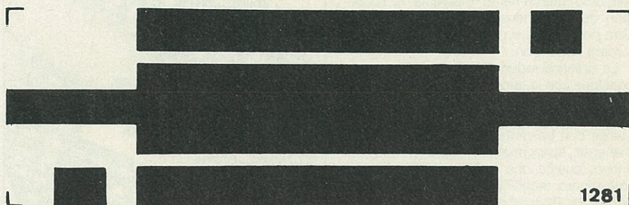
Figura 2. Plantilla del circuito impreso de las pistas de captación del medidor a tamaño 1:1.
