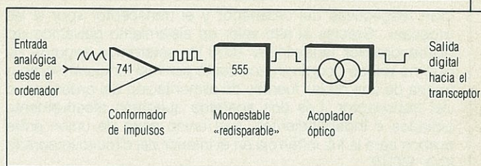
Figura 5. Esquema de principio del circuito anticlic.
