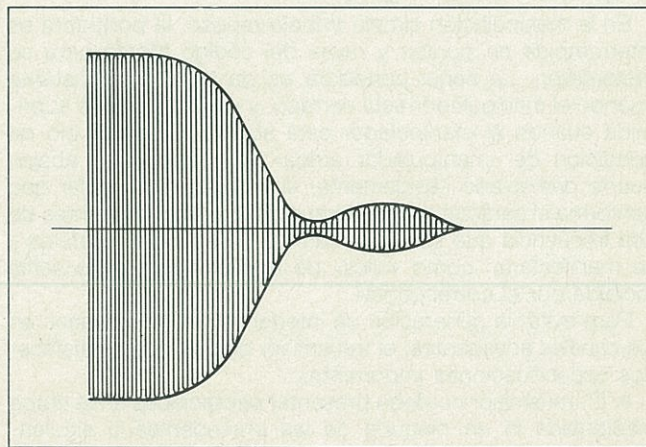
Figura 3. Entrando al transceptor por el conector de micrófono (AFSK), es casi seguro sobremodular la portadora y obtener una envolvente de RF como la mostrada en la figura, con numerosas bandas laterales.
