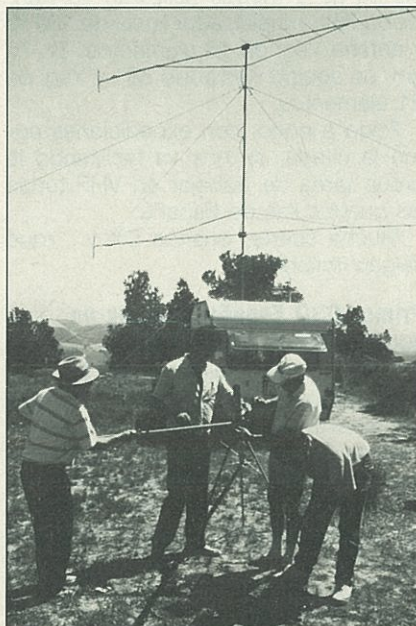
Preparando la antena de 432 MHz.
