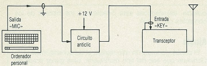
Figura 4. El circuito anticlic adapta las señales entre el ordenador y el transceptor.
