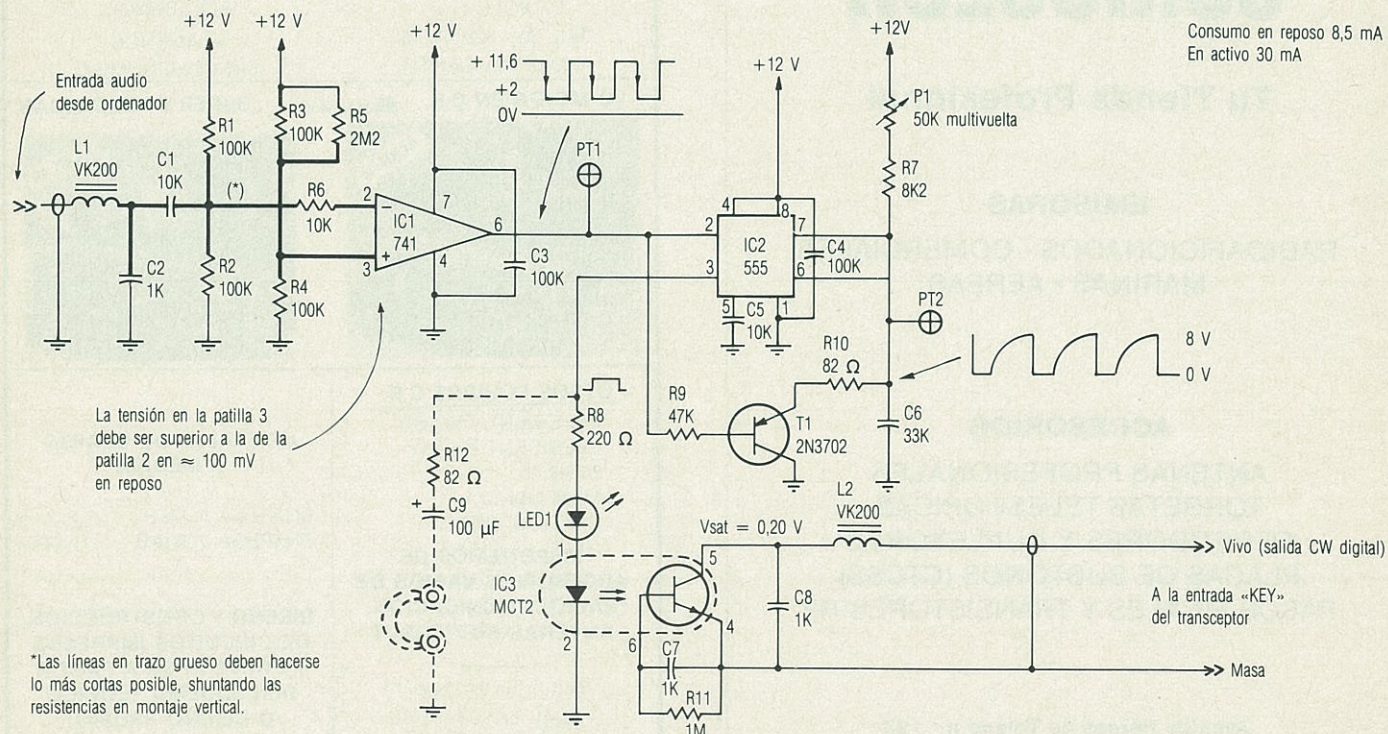
Figura 6. Esquema detallado del circuito anticlic.
