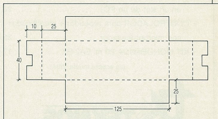
Figura 3. Desarrollo del blindaje del captador realizado en hojalata de 0,3 mm de grosor.
