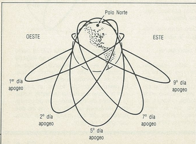
Ejemplo de las órbitas diarias del OSCAR 13 en un ciclo de diez días.
