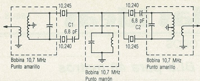
Figura 2. Filtro de cuarzo de construcción casera. C1 y C2 de unos 6,8 pF. Este valor actúa sobre el ancho de banda.
