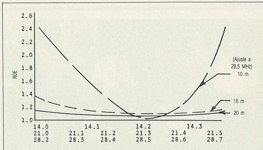
Figura 1. Curvas ROE facilitadas por el fabricante. Las nuestras resultaron muy parecidas.
