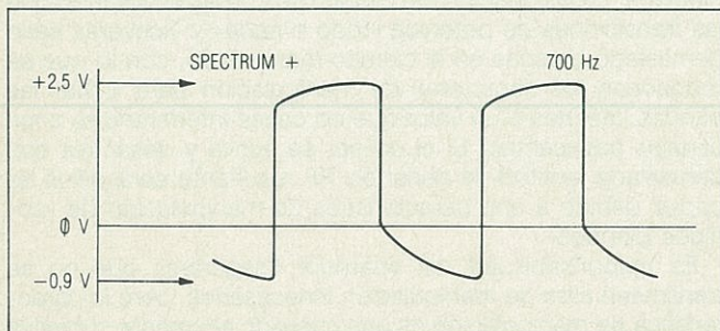
Figura 2. Forma de onda típica de la señal de audio entregada por el ordenador con el programa de CW cargado en su memoria.
