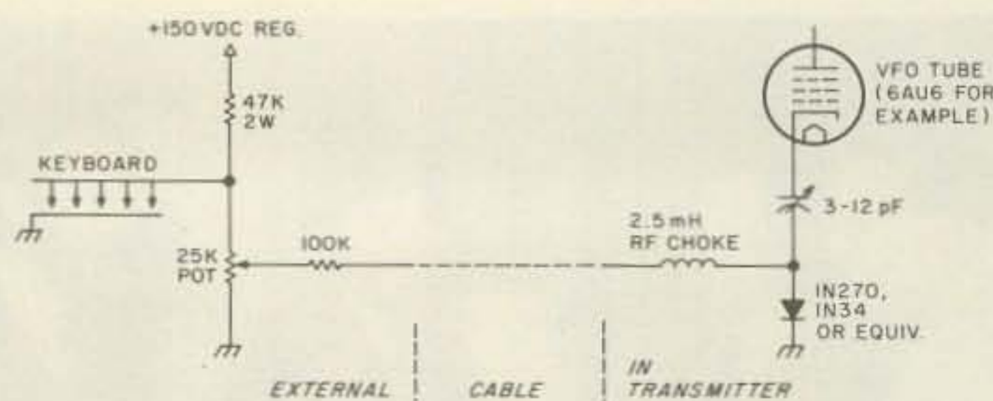
Fig. 2. Shift-pot circuit.
