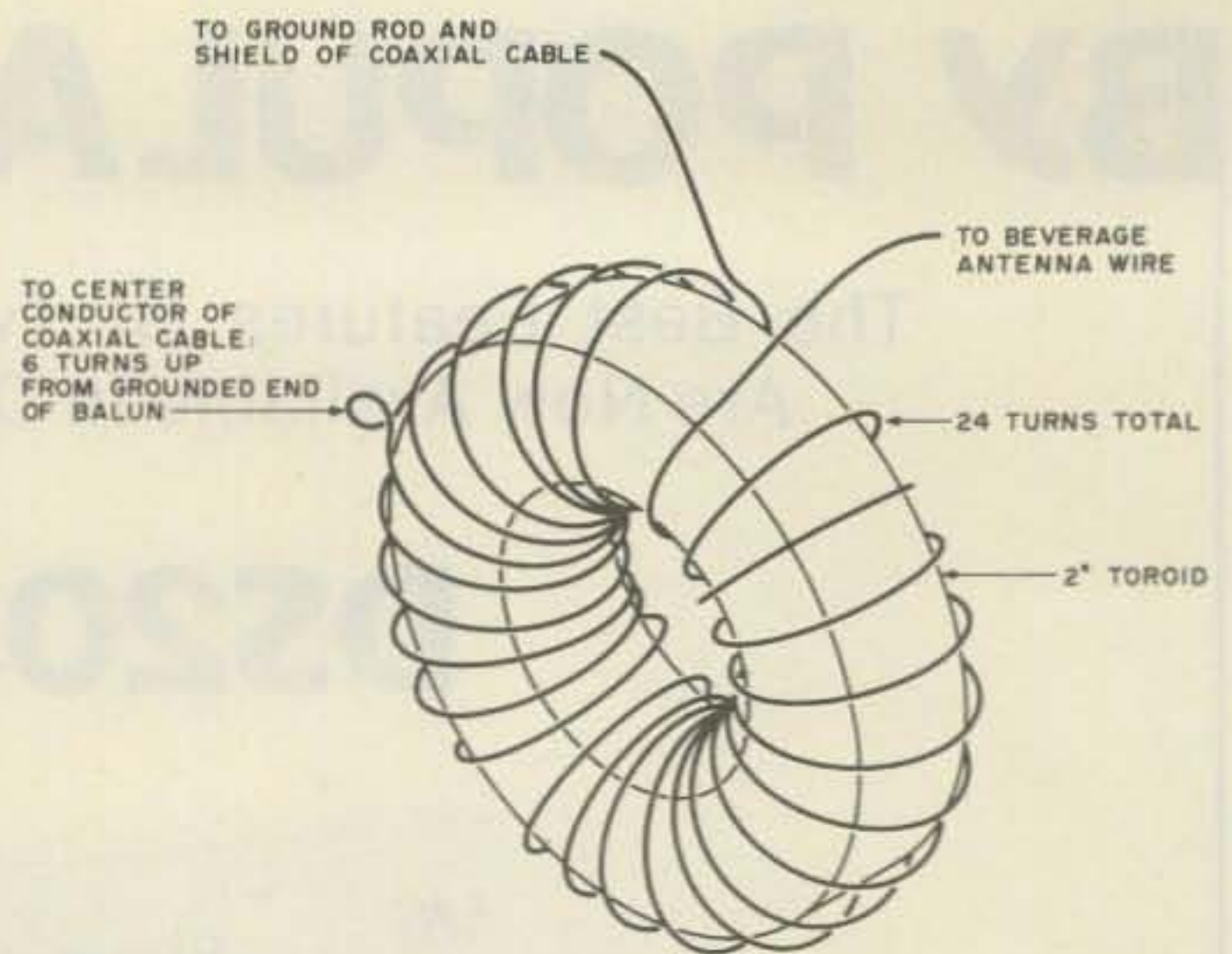
Fig. 2. A homemade 4:1 balun.
