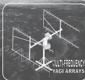
AE1000 SERIES AZ EL PEDESTAL
