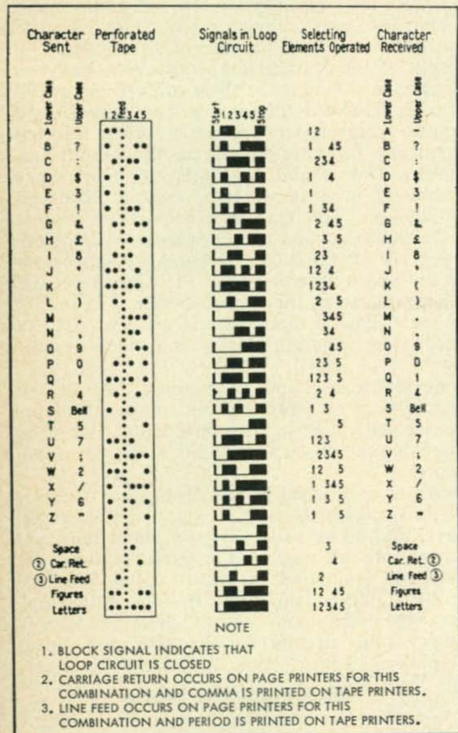
Fig. 1—Teletype Code
