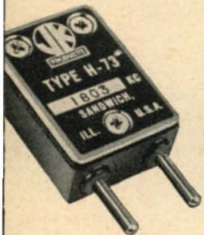
H-73 or H-7 (FT-243). Pin Dia. .090". Pin Spacing .500".
