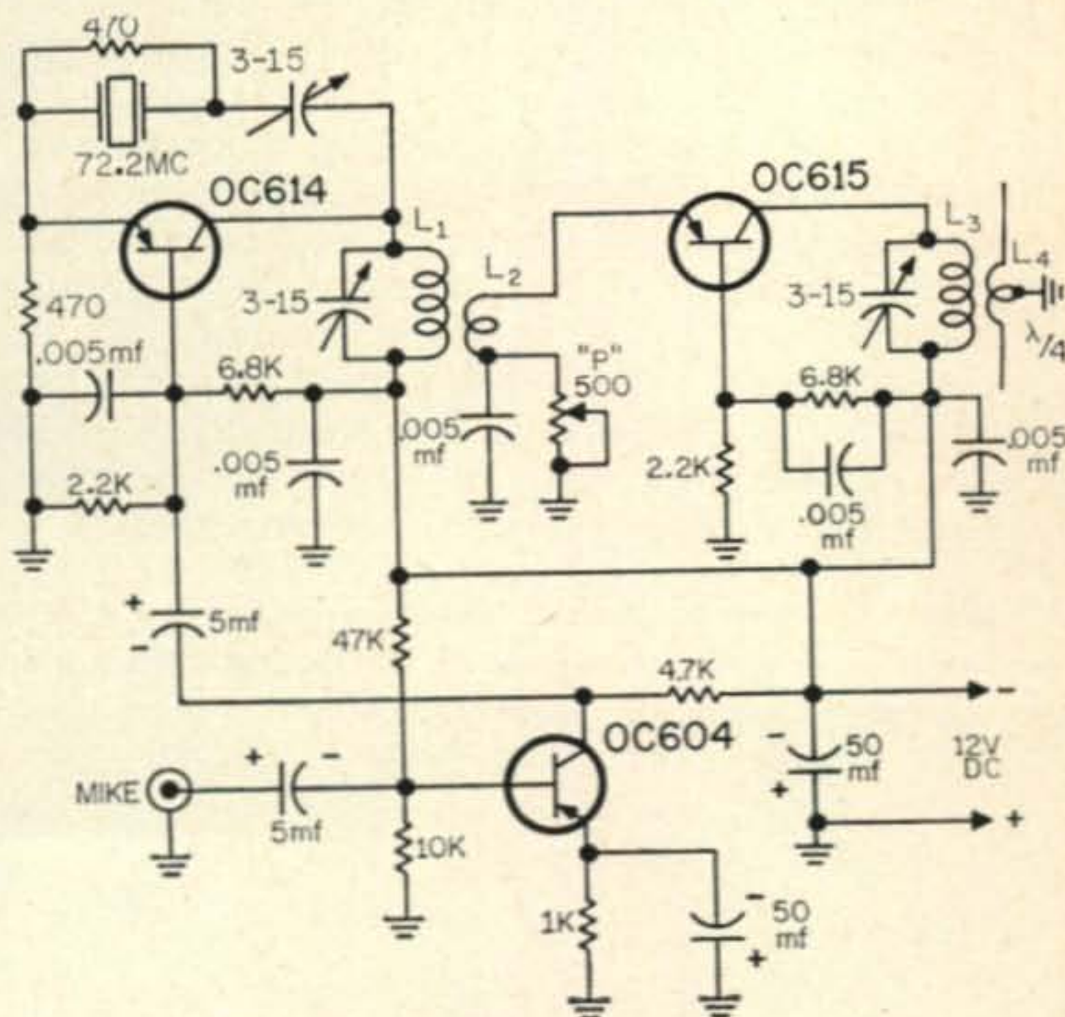
Fig. 3—Two meter transmitter.
