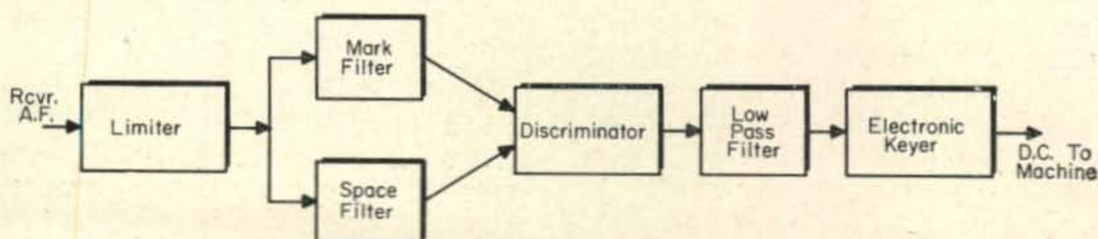
Fig. 4 A. F. FM converter block diagram.
