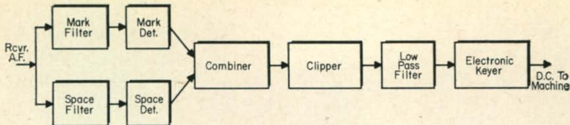
Fig. 5 A. F. filter converter block diagram.
