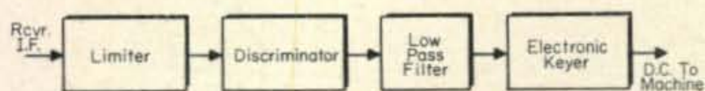
Fig. 3 I. F. converter block diagram.
