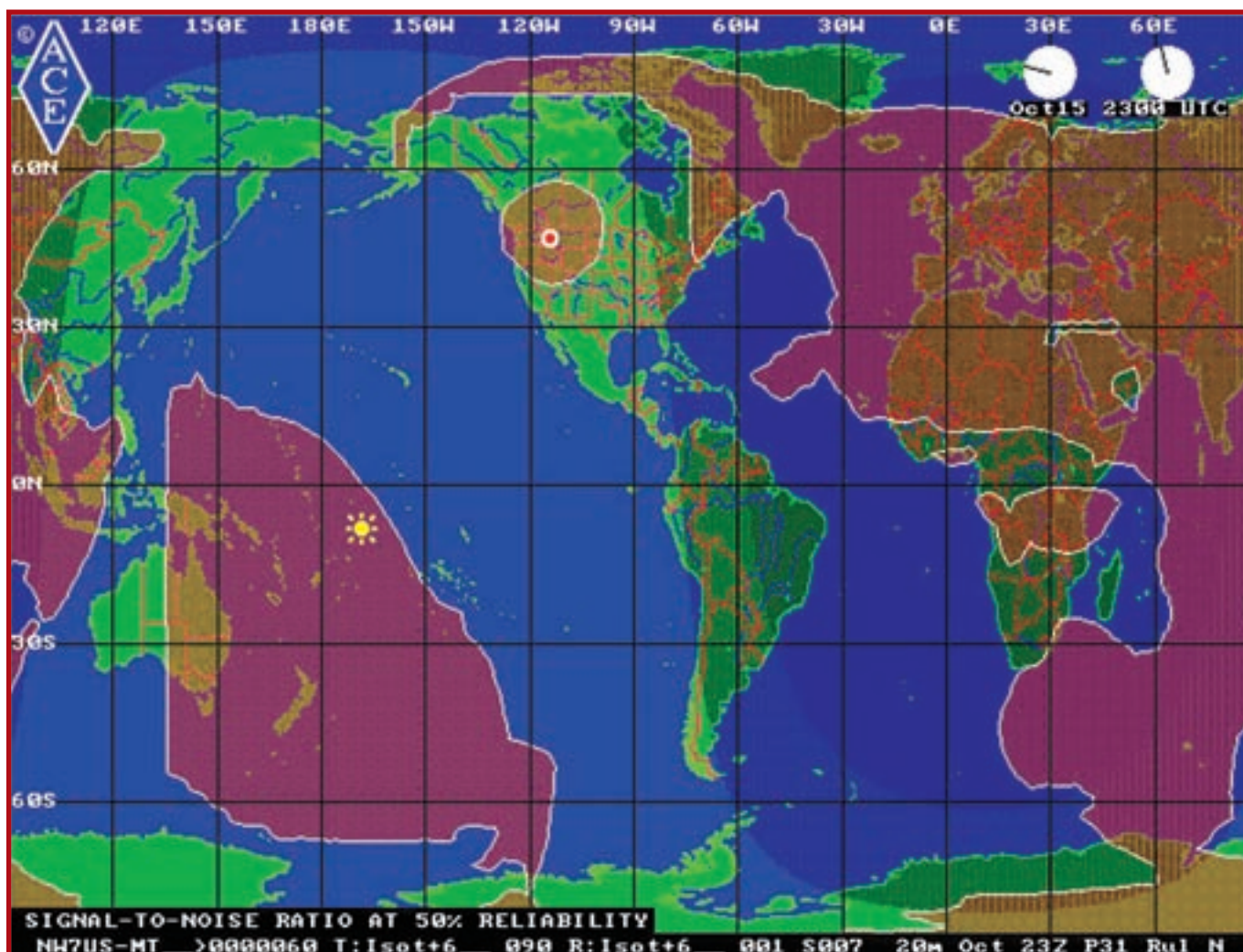
Figura 4. Mapa de cobertura de señal del programa ACE-HF Pro para las 2300 UTC de un día de octubre 2009, para una señal de 100 W en modo PSK-31 sobre una antena dipolo, desde el QTH de NW7US, en Montana. El mapa predice dónde puede ser recibida la señal durante la mitad de los días del mes. El área cubierta comprende la Antártida, como efectivamente se cumplió, con un QSO con DQ1POL. (Fuente: NW7US < http://hfradio.org/ace-hf >)
