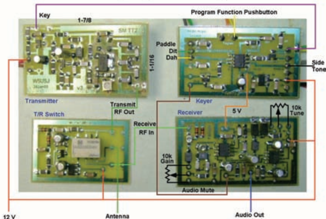
Foto G. Una vista más detallada de los cuatro módulos que completan el transceptor W5SUJ nos revelan que está compuesto por un transmisor Tuna-Tin 2 , un receptor MRX modificado, un manipulador Jackson Harbor y una placa de conmutación T/R similar a las utilizadas en el kit Tuna Tooper que proporciona < www.qrpme.com >. Chuck también ha grabado sus propias placas.
