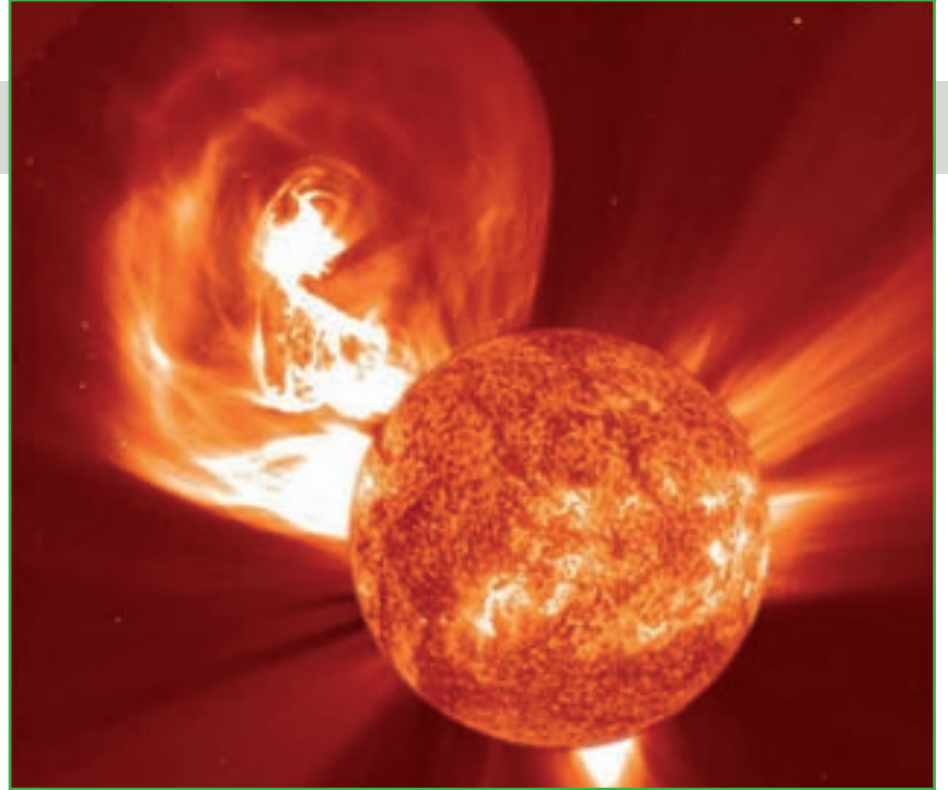
Figura 2: Impresionante imagen de una enorme eyección de masa coronal (CME) ocurrida el 4 de enero de 2002. Esta explosión expulsó miles de millones de toneladas de materia solar al espacio a velocidades de millones de kilómetros por hora. A las pocas horas se produjeron severas anomalías en la propagación por radio en la Tierra. Fuente: NASA
