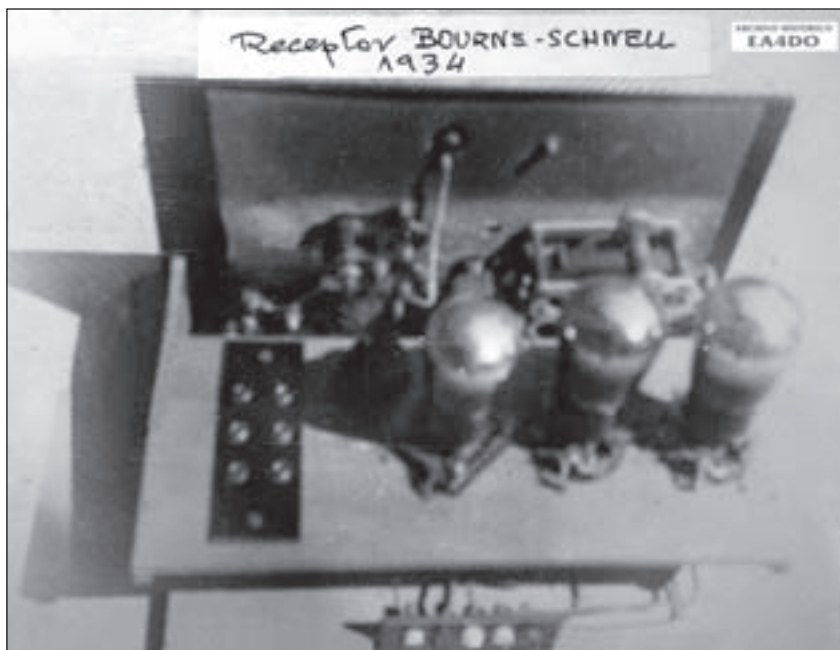
Foto B. Vista del receptor regenerativo tipo Bourne-Schnellen , usual entre los aficionados de pre-guerra. Aunque lo usual era equiparlos con sólo dos válvulas, una como detector regenerativo y otra como amplificadora de B.F., en este modelo aparece una tercera válvula, supuestamente como amplificadora final de audio.
