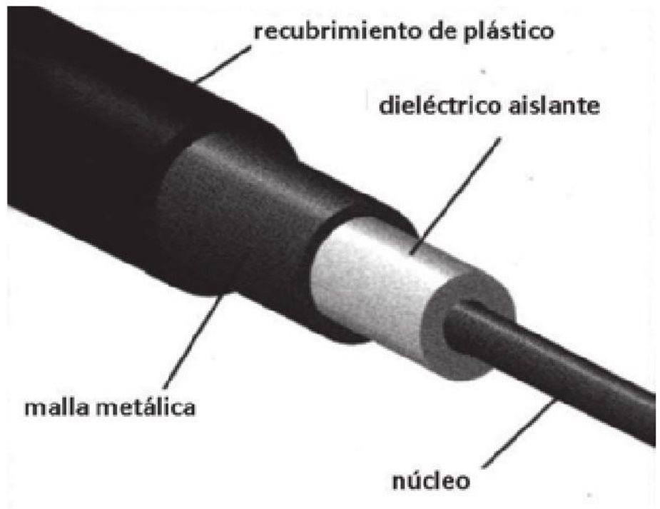
Foto A: Corte de un cable coaxial (Foto cedida por Wikimedia Commons, bajo licencia Creative Commons ( http://creativecommons.org/licenses/by3.0/deed.en ))
