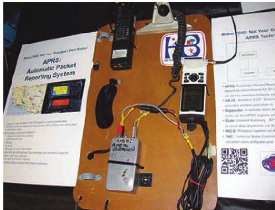
Figura 4: La baliza de APRS de KH6WZ consistía en un viejo equipo de 2 metro, una TNC TinyTrak2 de Byonics y un GPS de Garmin. Es estupendo que aún funcione este conjunto que tiene ya más de 10 años.
