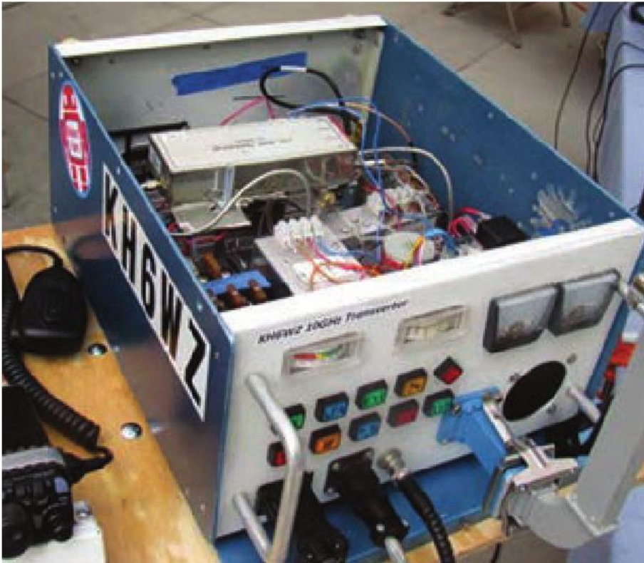
Figura 5: Mi sistema de transverores de 10 GHz, con la tapa quitada, se convirtió en una pieza importante de la exhibición. Un diagrama de bloques simplificado explicaba el funcionamiento de su interior y cómo funcionaban las mates de la multiplicación de frecuencia. Mi detector de microondas (el medidor de campo visible a la izquierda) fue utilizado para demostrar la polarización, la ganancia y el diagrama de radiación de una antena y sus nulos.
