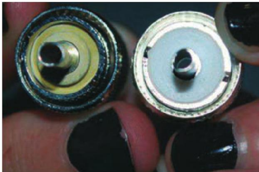
Foto D: Un par de conectores PL-259. El de la izquierda es un Amphenol. El de la derecha es uno más barato.
