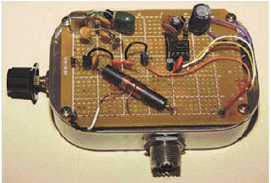
El receptor "Lata de sardinas" es un buen compañero para el clásico transmisor QRP Sardine para CW diseñado por W1FB.
