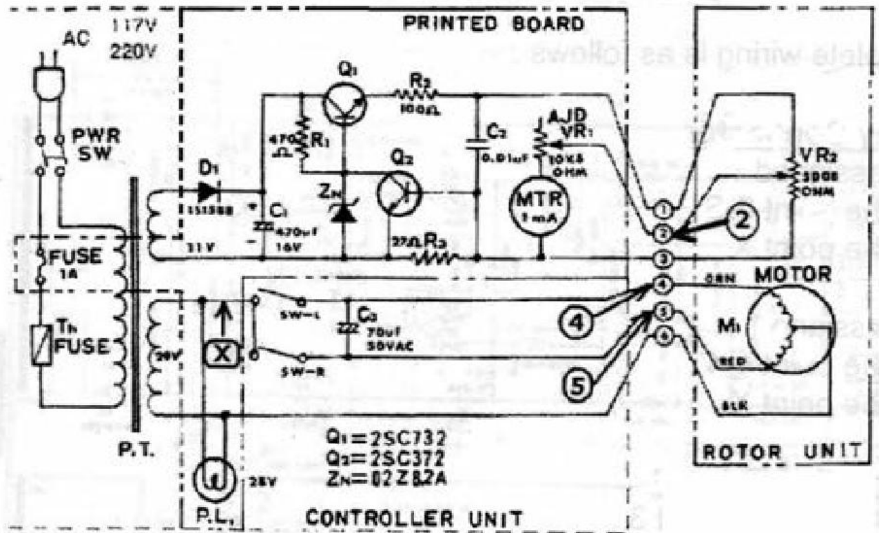
Figura 8 Esquema KR-500
