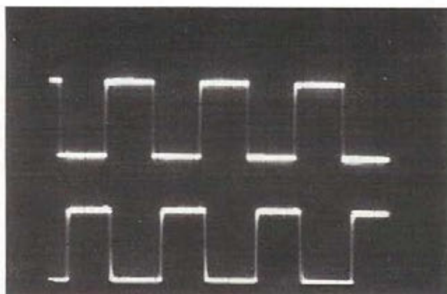
PHOTO 4: F_1 \cong F_0 + F_c Le déphasage entre V_1 et V_r atteint presque \pi . La valeur moyenne de V_1 , sortie du OU exclusif atteint V_{DD} .
