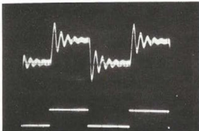
PHOTO 1 (0,5 ms/carreau): Réponse linéaire de la boucle (en haut) à un échelon de fréquence (en bas) D = \frac{a}{b} = 0,7 ; tr \cong 600 \mu s
