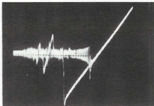
PHOTO 6: Agrandissement de la précédente, le balayage n'atteignant plus F_0 + F_i .
