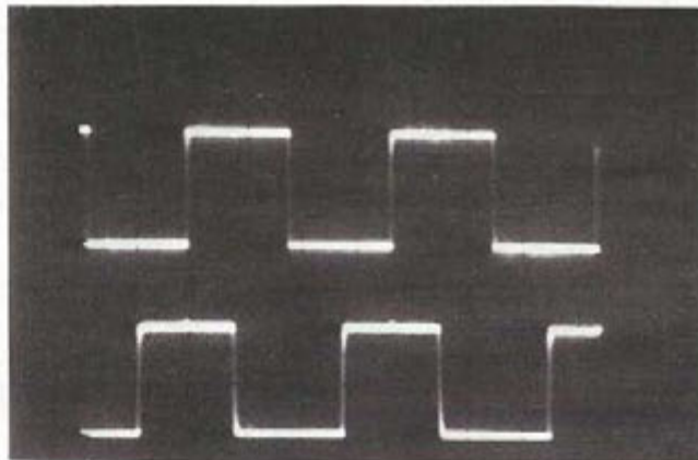
PHOTO 2: F_1 \cong F_0 . La valeur moyenne de V_1 vaut 0,5 V_{DD} V_1 en bas V_r en haut 5V/cm 5 \mu s /carreau Il y a un déphasage de \pi/2 entre V_1 et V_r .
