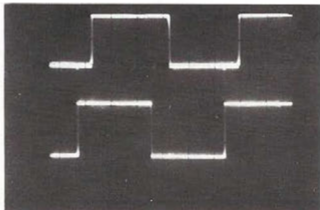
PHOTO 3: mêmes légendes que la photo 2. Ici F_1 \cong F_0 - F_c . Il y a un déphasage presque nul entre V_1 et V_r . La valeur moyenne de V_1 est presque nulle.
