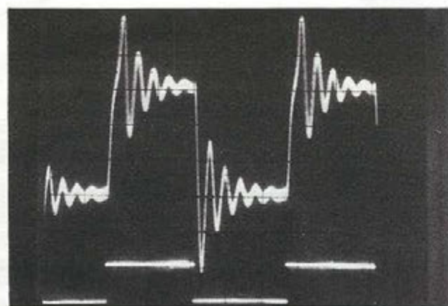
PHOTO 7: F_i proche de F_0 + F_c .
