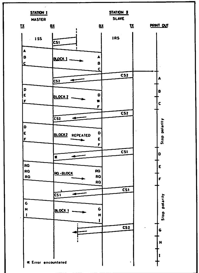
ARQ - AVEC CONDITION ERREUR
