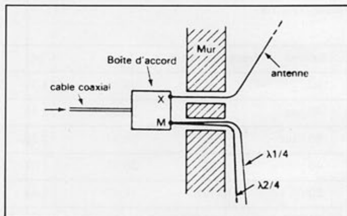
Figure IV.2.11e. - Si l'on doit utiliser des radians uniques placés à l'extérieur, ils seront installés dans des directions les plus opposées possibles à celle de l'antenne.
