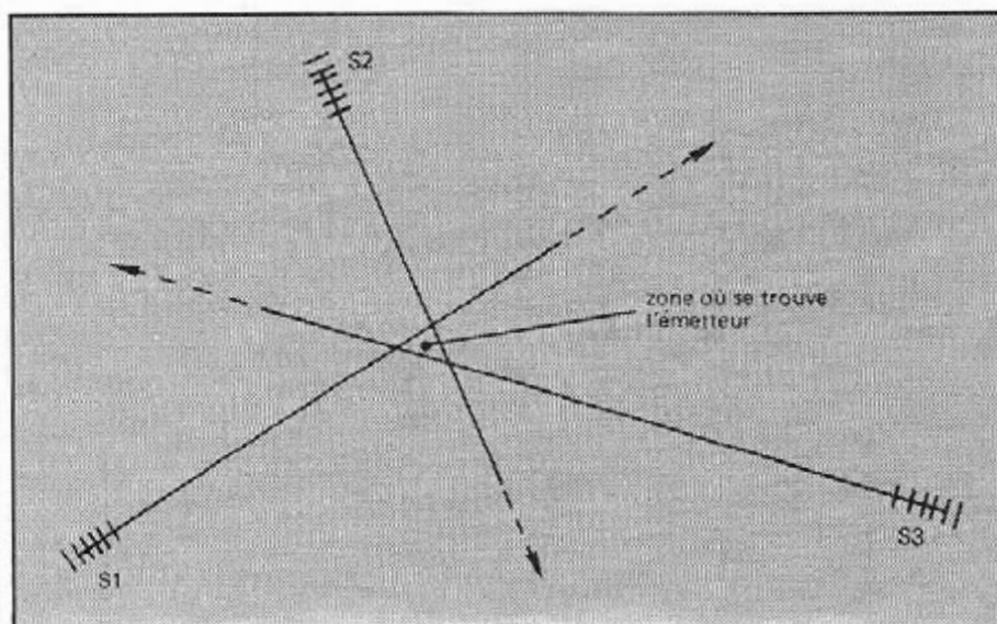
Figure 1 Avec trois stations on obtient un triangle dans lequel se trouve l'émetteur recherché, d'où le nom de triangulation.
