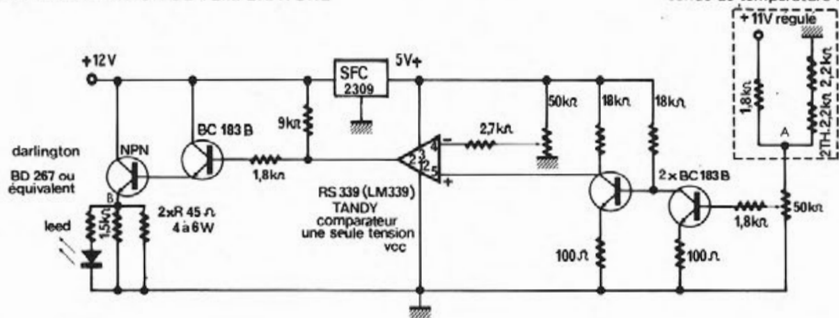
sonde de température interne
