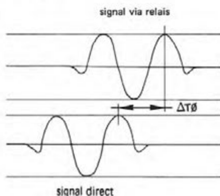
Figure 5 Mesure de \Delta T_0 sur des trains de sinusoïdes BF.
