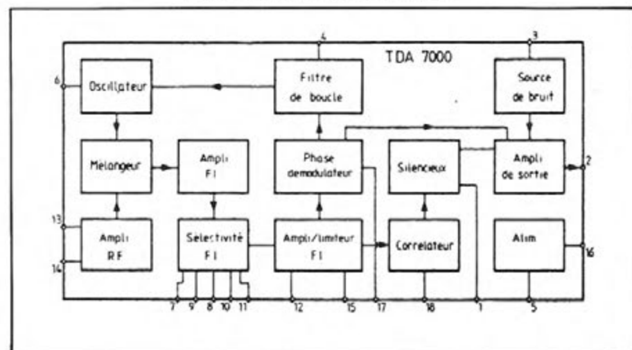
Figure 1 : Synoptique du TDA 7000
