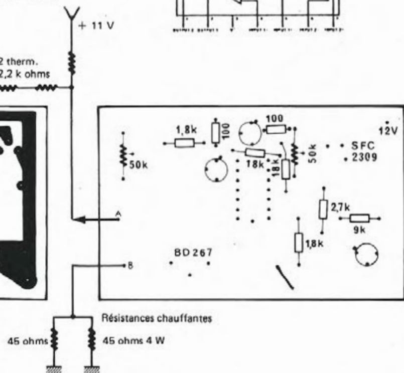
sonde de température interne
