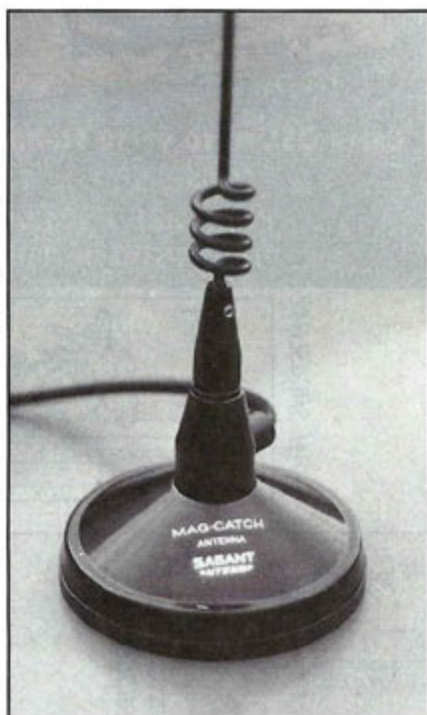
Détail de la self et de l'embase magnétique.
