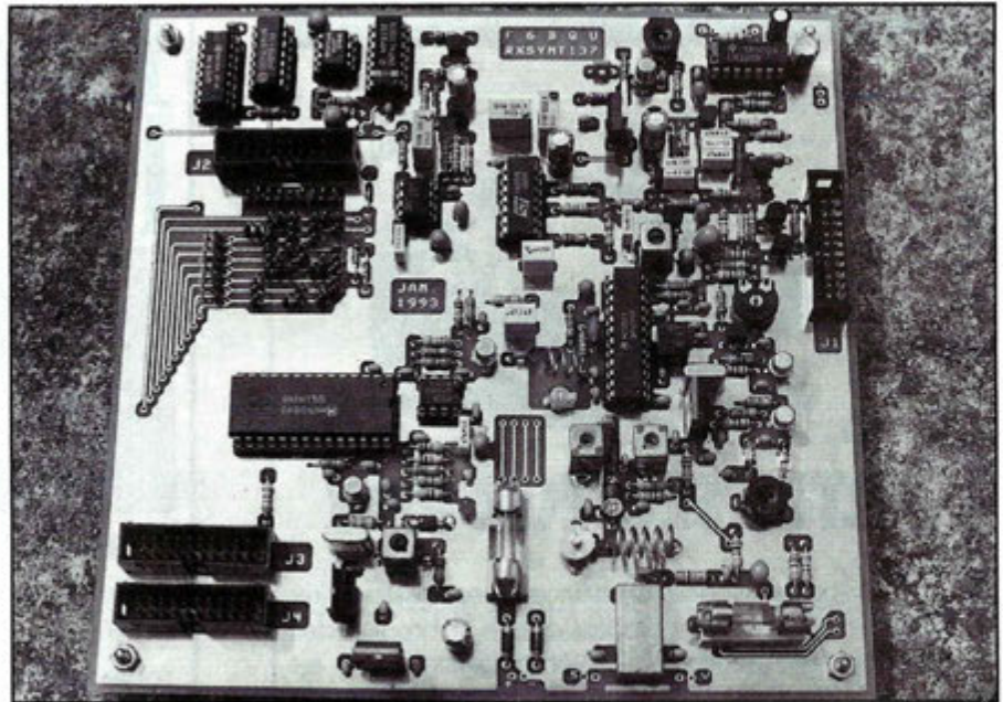
Vue des composants sur le circuit imprimé
