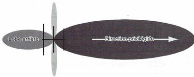
Figure 2 : Lobe de rayonnement théorique d'une antenne Yagi.
