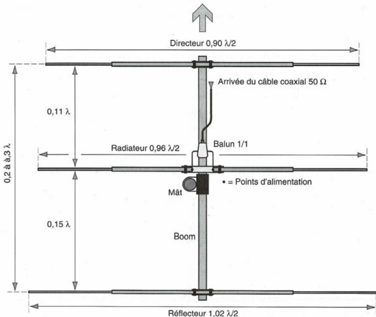
Figure 3 : Réalisation d'une Yagi 3 éléments.
