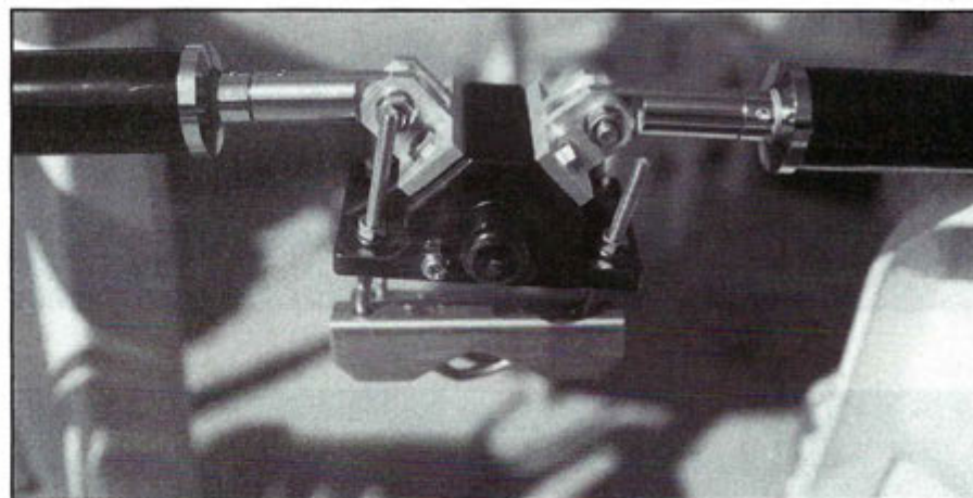
Vu de l'antenne au niveau de la fixation et de l'alimentation.
