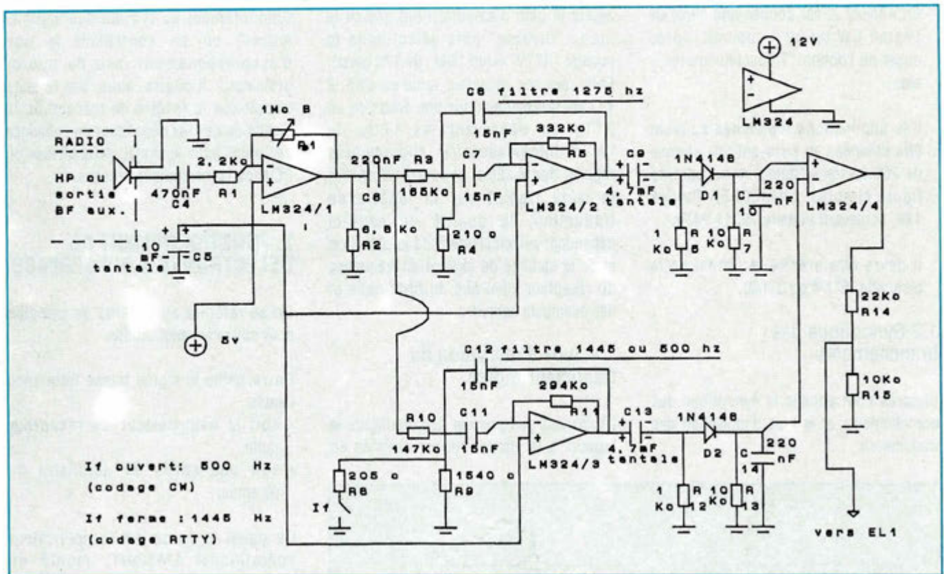
SCHEMA DE PRINCIPE - PARTIE ANALOGIQUE
