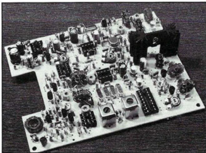
La platine finie.
