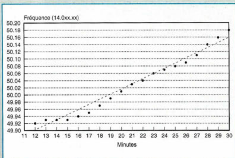
Dérive du VFO.
