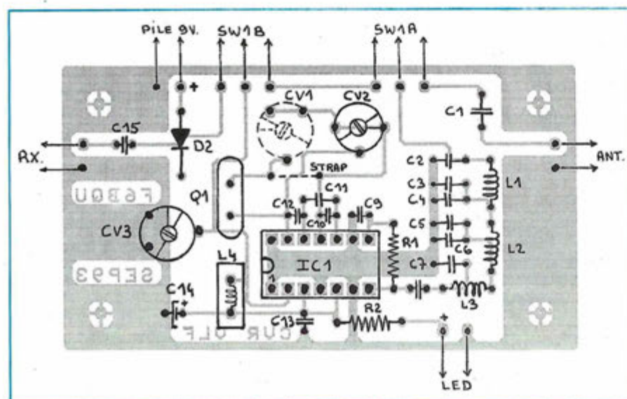
Schéma d'implantation.
