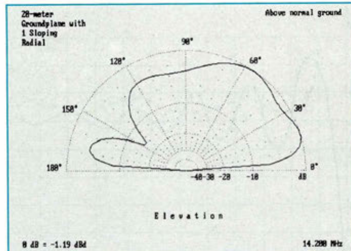
Figure 6. Diagramme vertical d'une "GP1RAD" 20 m située au-dessus du sol.
