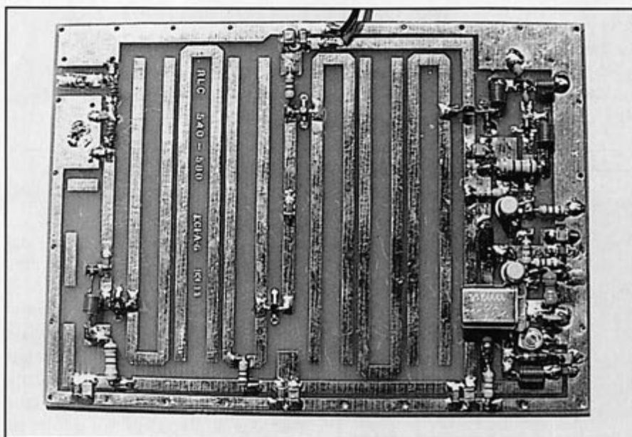
La carte SHF-LO (Oscillateur local) identique sur les deux transverters.
