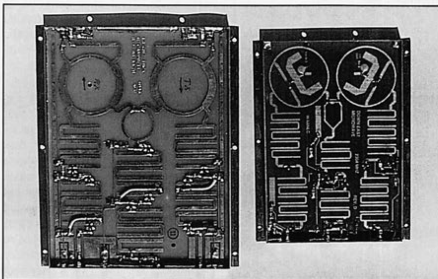
Les deux cartes des mélangeurs : - La grande pour le 23 cm - La petite pour le 13 cm.
