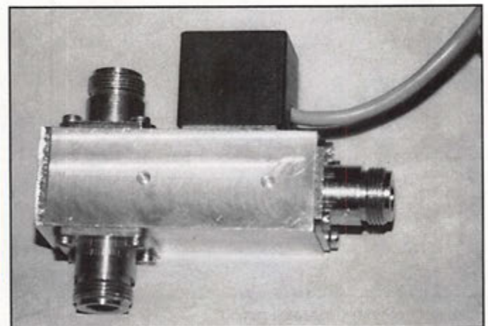
Le relais VHF/UHF tel que vous le construirez dans la seconde partie de l'article.
