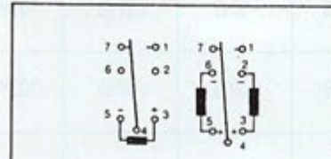
A) Relais monostable: raccordez le contact 1,4 se ferme
