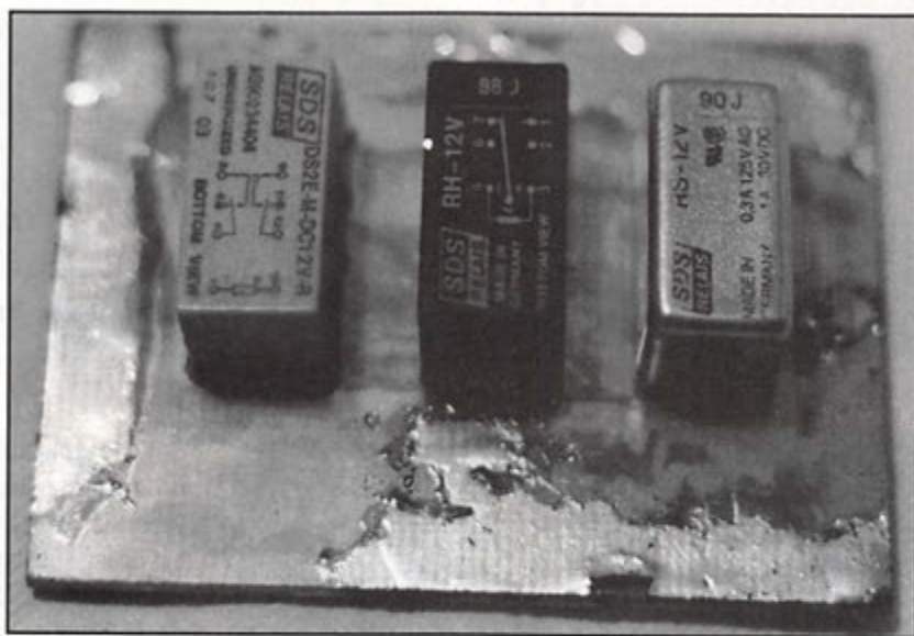
Photo de la platine ayant servi aux mesures sur les petits relais.
