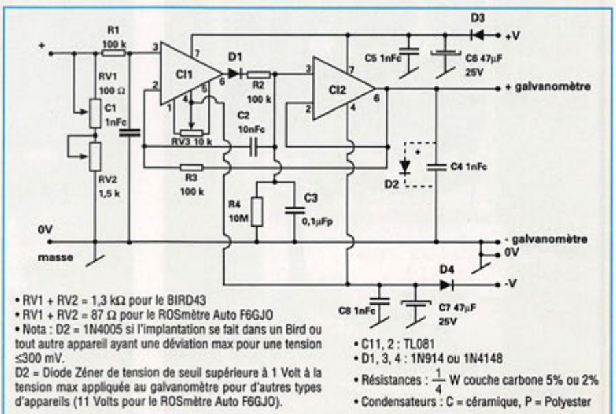
Figure 4 - Schéma.
