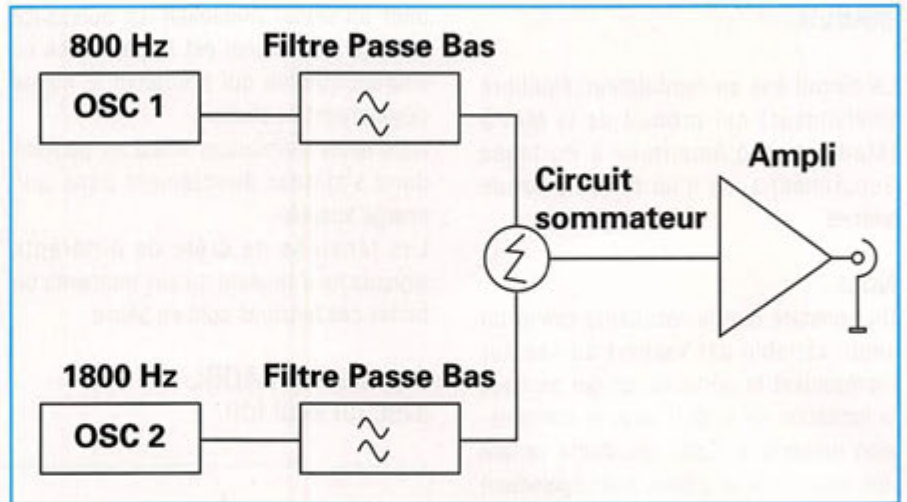
Figure 1 - Synoptique d'un générateur deux tons.
