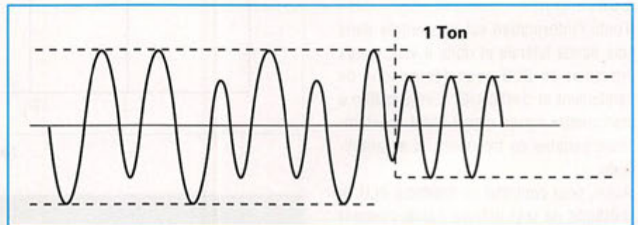
Figure 2 - Allure du signal deux tons.
