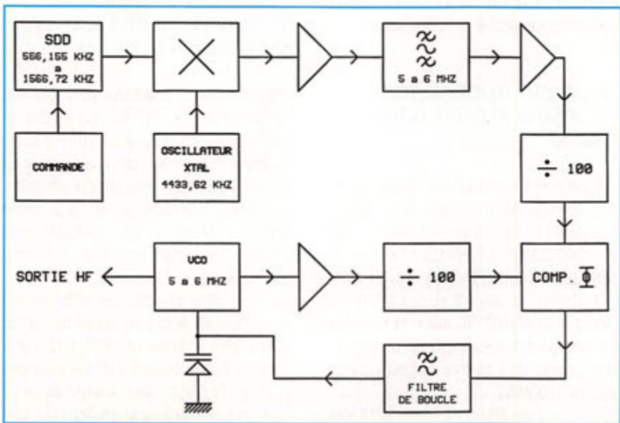
Fig. 1 - Diagramme fonctionnel.
