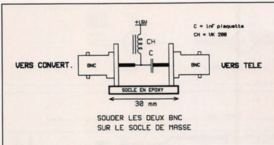
Alimentation du convertisseur via le câble coaxial
