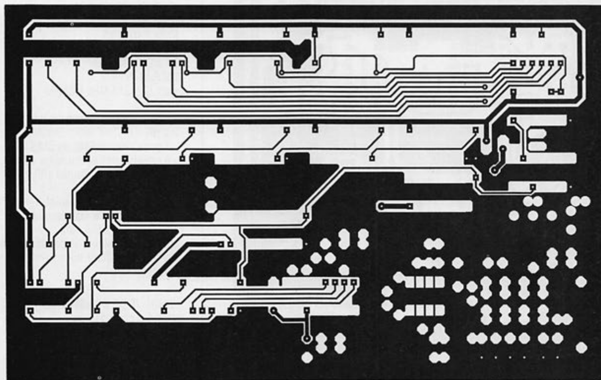
SYNTHESE DIGITALE DIRECTE :côté composants.
