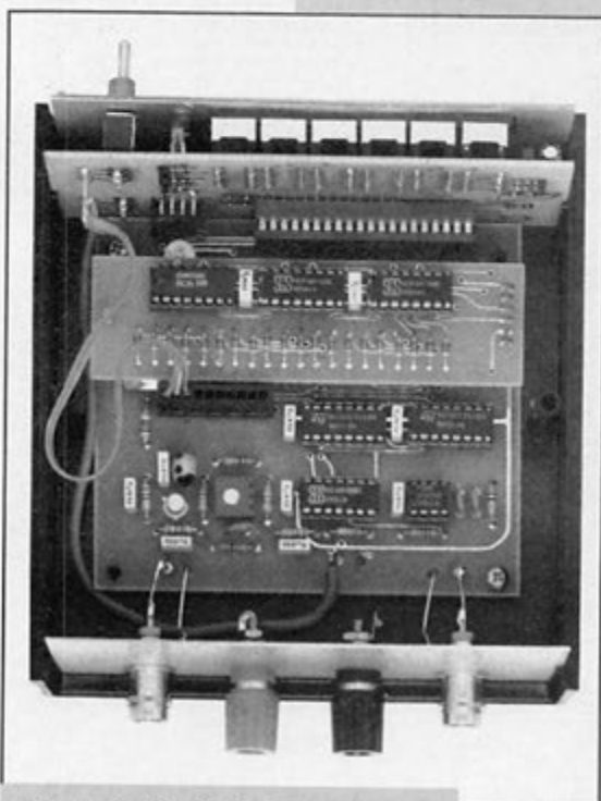
Photo 2. Vue intérieure.
