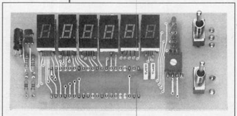
Photo 5b. Le circuit d'affichage.
