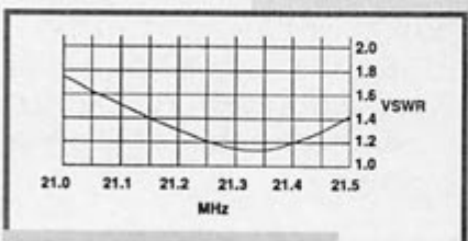
Courbe 5.
