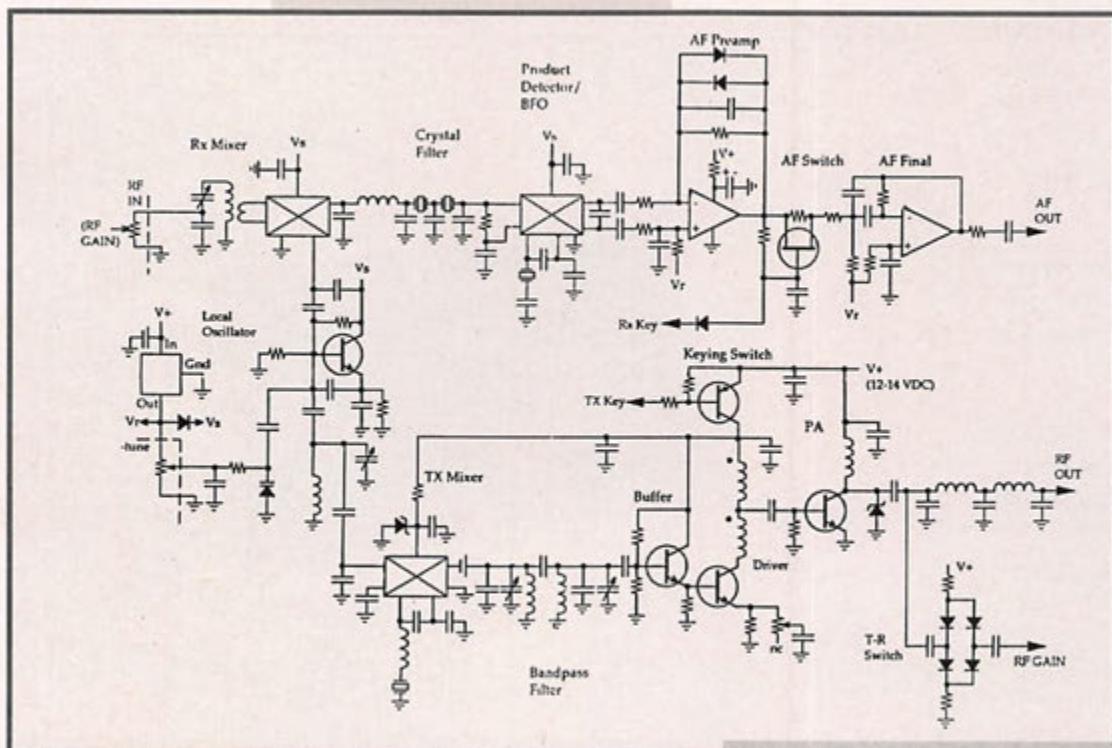
Schéma électronique.
