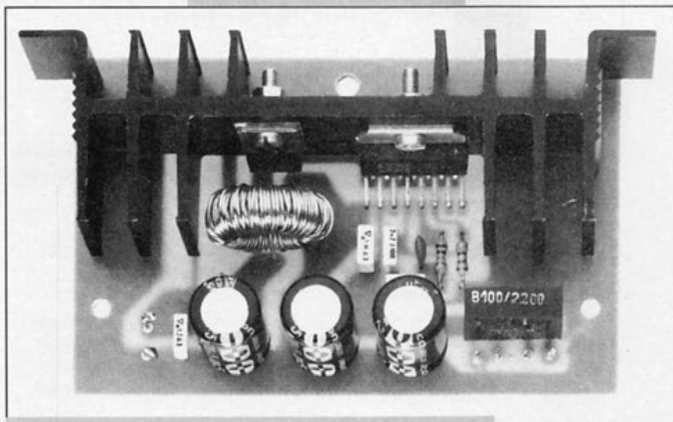
Photo 6. L'alimentation.
