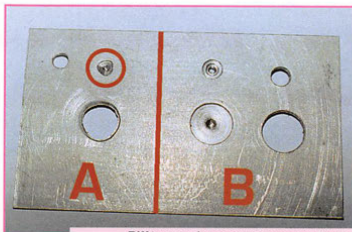
Différence de perçage entre un foret classique Rep.A et un foret modifié Rep. B.
