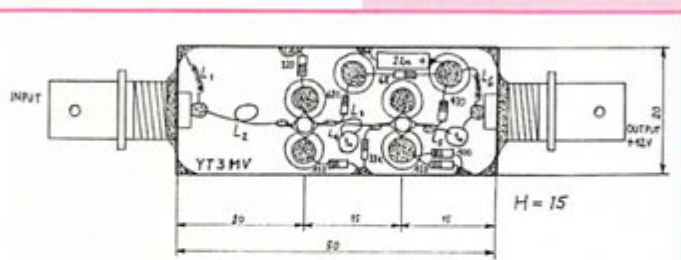
Figure 2 : Croquis du préampli YT3MV avec implantation des composants.
