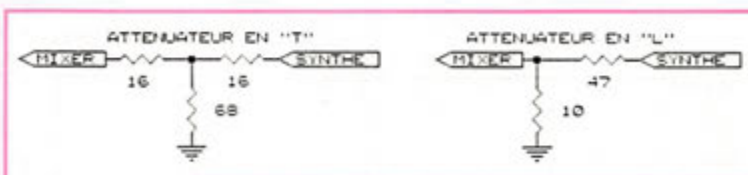
Figure 6 : Atténuateurs pour le récepteur.
