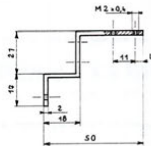
Désignation : support vis marteau Rep : ⑦ Nbre : 2 Matière : Cu Zn 15 Echelle : 1
