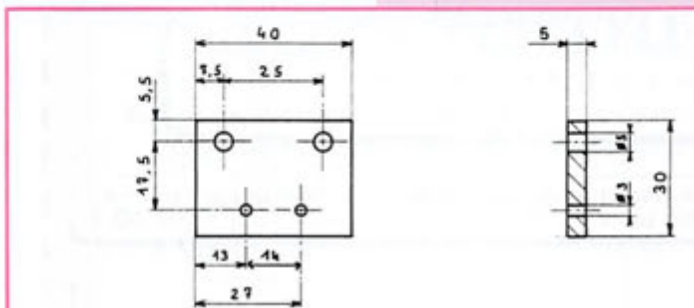
Désignation : plaque supérieure de maintien d'axe de basculeur Rep : ⑤ Nbre : 1 Matière : AU4G Echelle : 1
