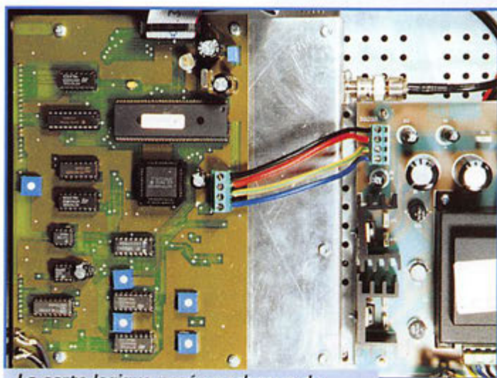
La carte logique posée au-dessus du boîtier blindé contenant les circuits HF.
