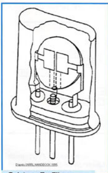
Schéma 5: Filtre monolithique.
