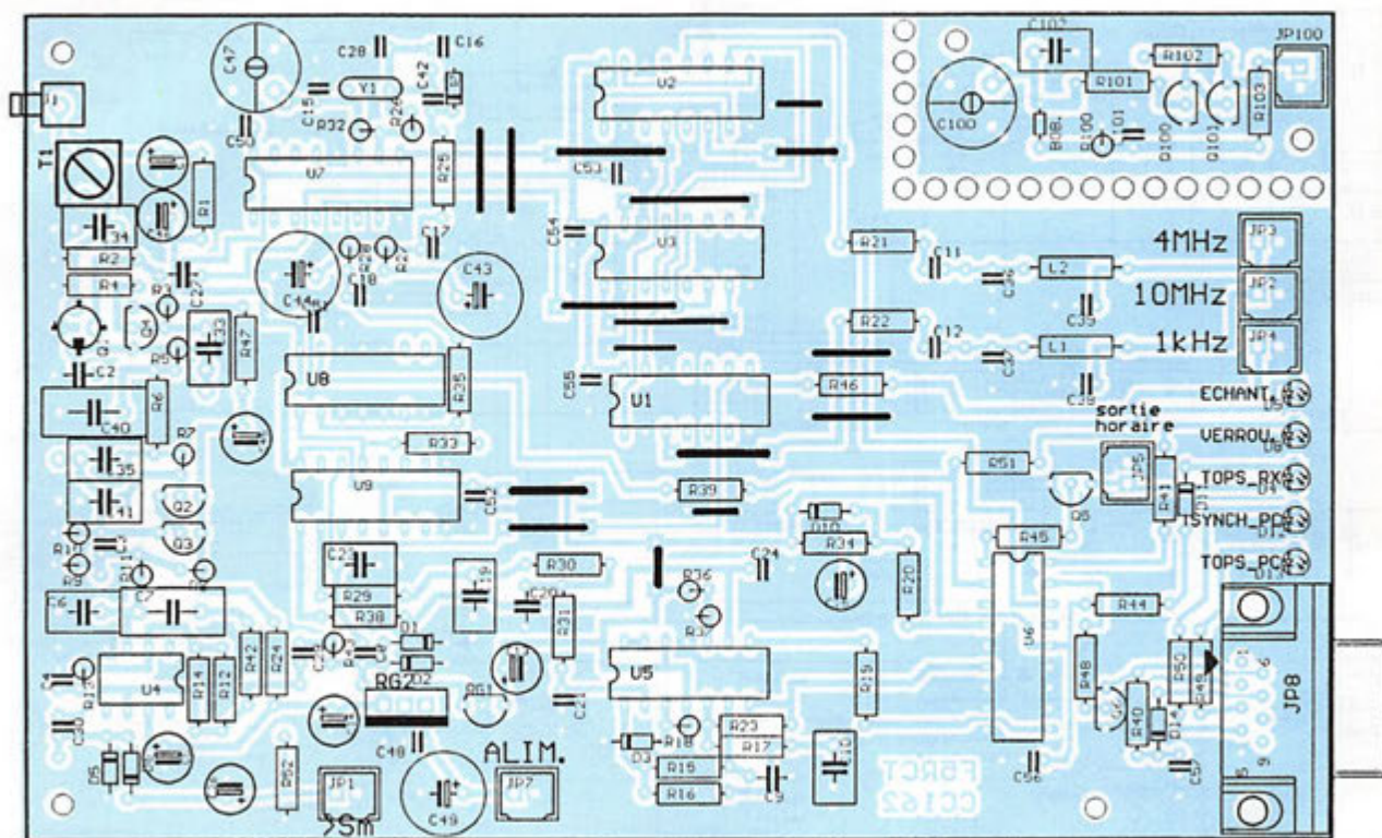
Implantation des composants.
