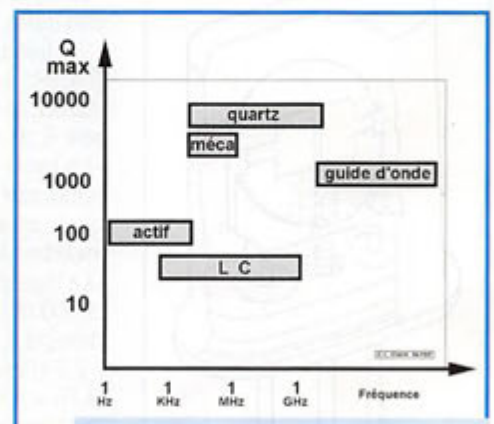
Schéma 3 : Fréquence d'utilisation et Q maximum de filtres passe-bande selon la technique employée.
