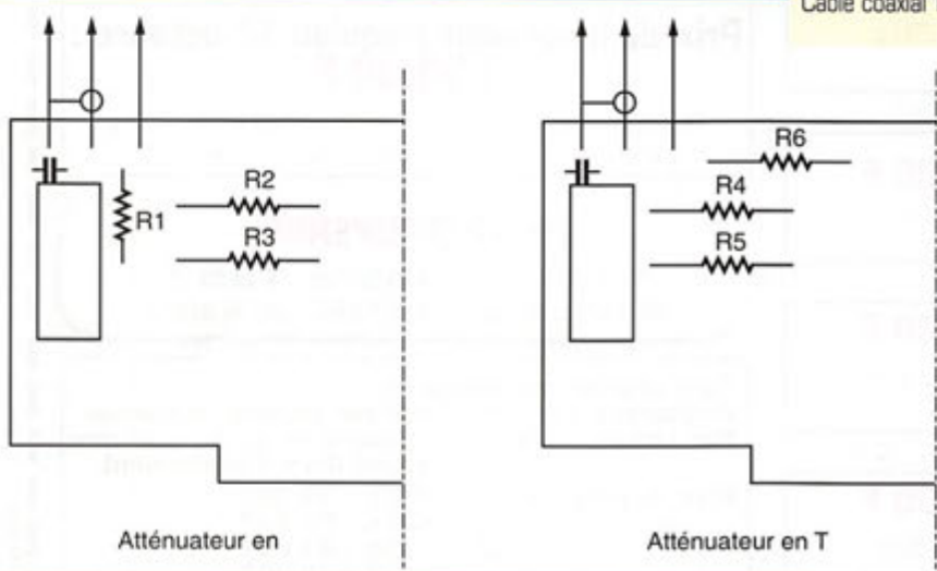
Implantation des résistances de l'atténuateur.
