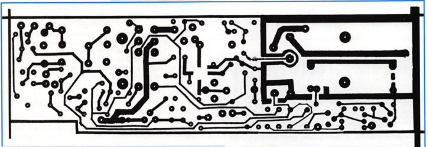
Circuit imprimé côté soudures.
