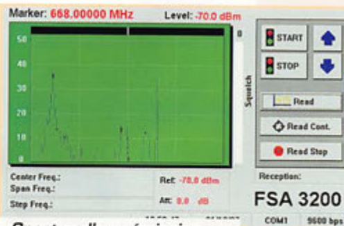
Spectre d'une émission TV.
