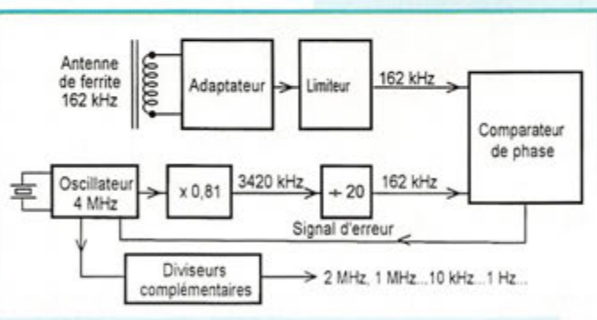
Fig. 1. — Dans le récepteur de fréquence étalon, un oscillateur à quartz de 4 MHz se trouve asservi, notamment au moyen d'un multiplicateur de rapport, à la porteuse de France Inter, 162 kHz.
