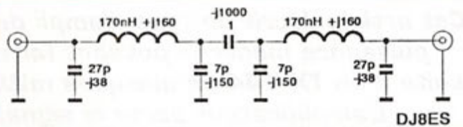
Fig. 5 : Filtre passe-bas.
