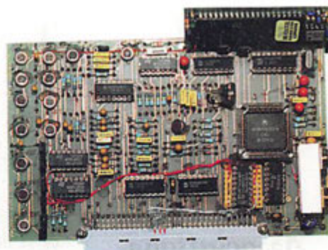
Carte logique principale : gestion relais PTT, CTCSS, BF, 1750.
