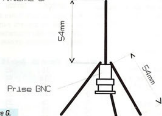
Antenne GP
