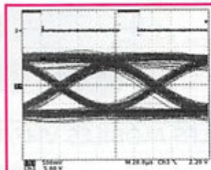
Diagramme de l'œil normal.
