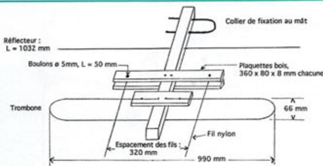
Fig. 2. Côté trombone : Le directeur, la plaquette de maintien de distance entre les fils, et le trombone sont montés sur une partie rigide fixée au mât. L'autre extrémité de l'antenne ne comporte que les plaquettes d'espacement.
