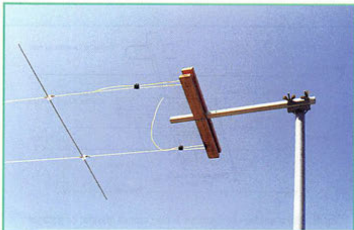
Le 18e brin-directeur à l'autre extrémité de l'antenne, et le support des fils. Les dominos permettent le réglage précis des longueurs de fil nylon.
