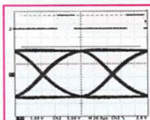
Diagramme de l'œil en émission.
