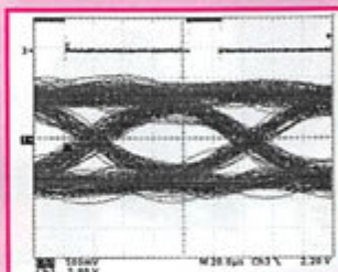
Diagramme de l'œil avec du bruit.
