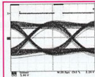
Diagramme de l'œil avec amplification des fréquences hautes.
