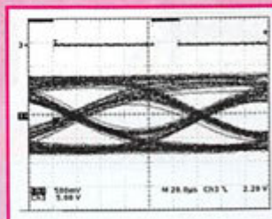
Diagramme de l'œil avec atténuation des fréquences hautes.
