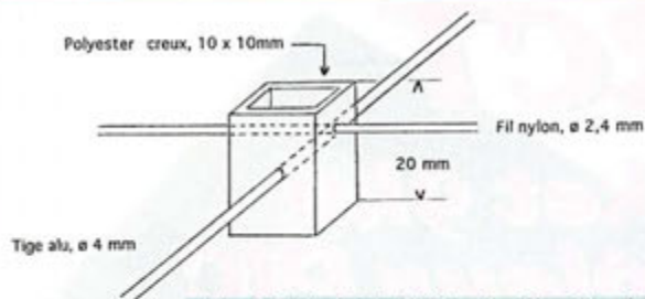
Fig. 4. Solidification fil-éléments : Une pièce de liaison, ici en polyester, est percée de deux trous à 90°, l'ensemble est ensuite fixé à la colle.
