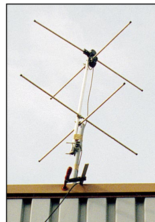
Antenne 137 MHz.
