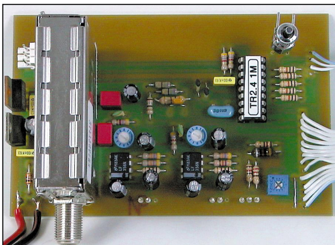
▼ Vue de la platine TX.
