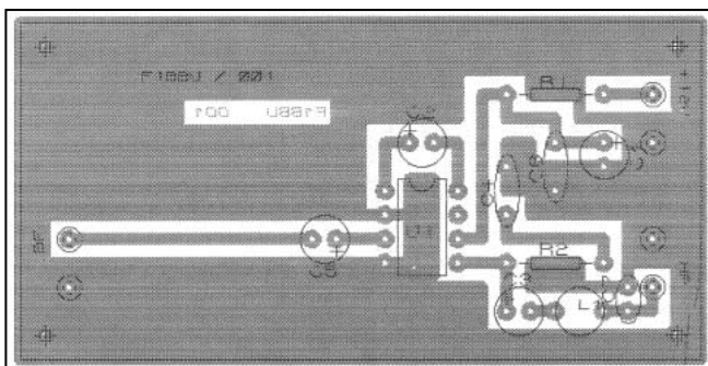
Implantation de l'ampli BF 300 mW.
