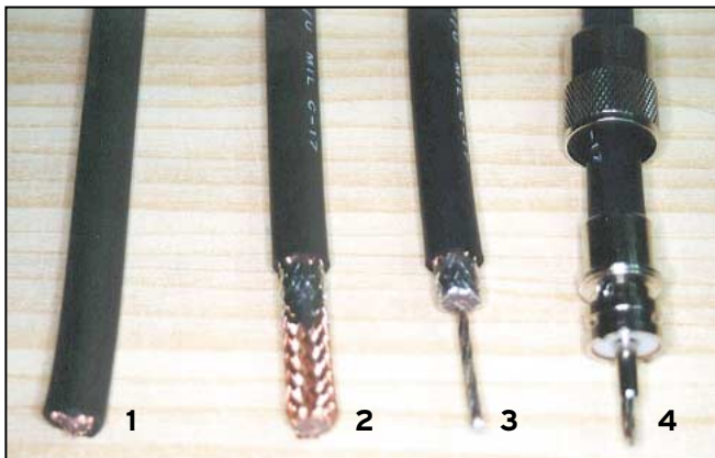
Figure 3 - Montage d'un connecteur PL-259.
