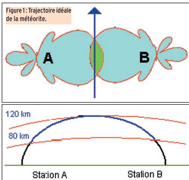
Figure 2 : Trajectoire tangente.
