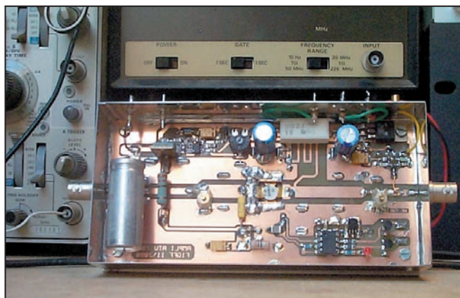
Ampli 3W.
