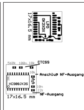
Figure 10 : Tracé du nouveau CI.
