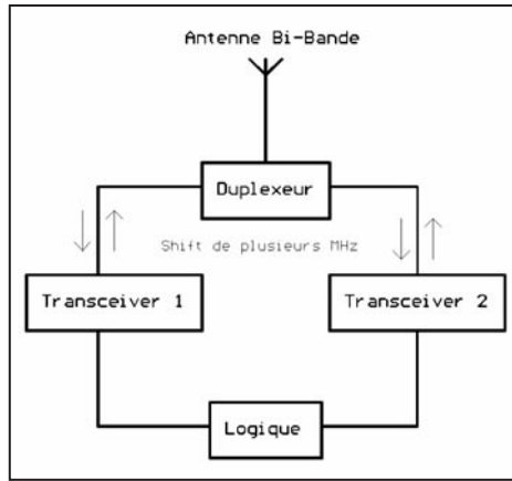
Relais transpondeur avec une antenne.
