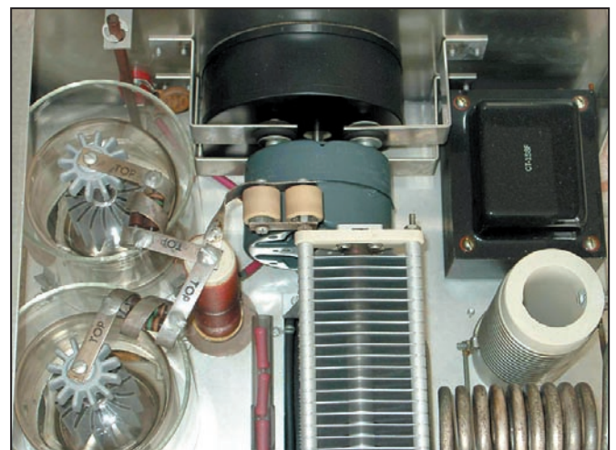
Vue intérieure du Drake L4B.
