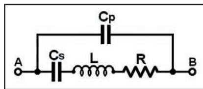
Figure 3: Schéma équivalent à un quartz.
