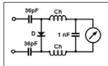
Figure 7: Schéma de l'appareil de mesure.
