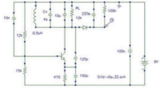
RL 1000k à 10k ; Vdc va de 9,5 V à 8,8V ( avec 0,5uH , 4 pF à 21 MHz ) RL 1000k à 10k ; Vdc va de 9,3V à 8,8V ( avec 0,5uH , 70pF à 17 MHz ) Spectre TRES sale , largeur de 0,7MHz à 50% d'amplitude @ 21 MHz
