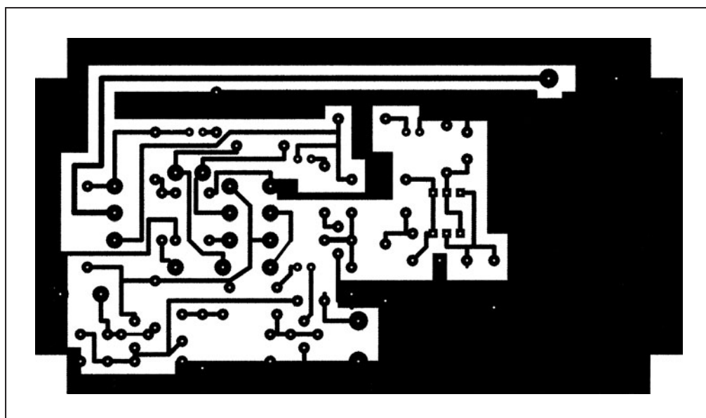
Figure 4: Dessin du circuit imprimé, à l'échelle 1, vu côté cuivre.
