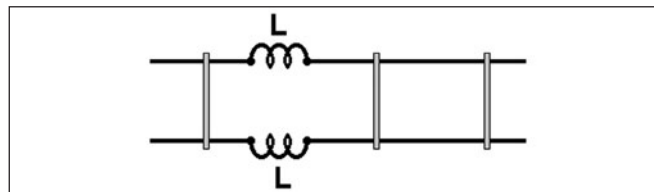
6 - Ligne allongée à l'aide de bobines.
