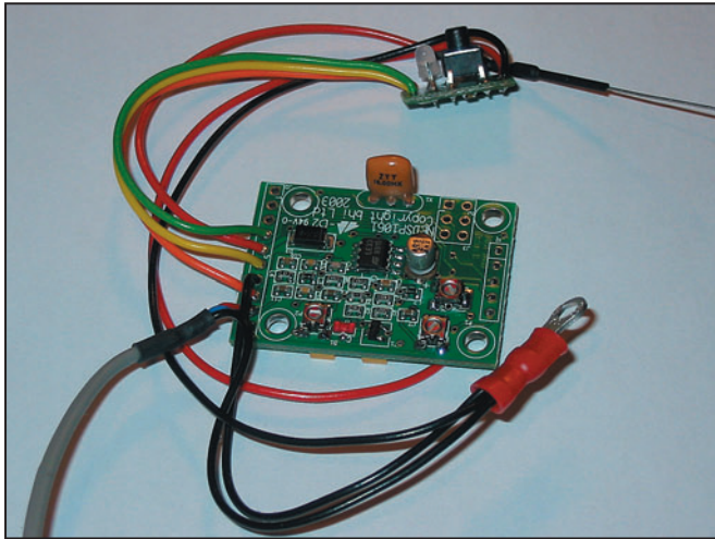
5 - Module DSP NEDSP1061-KBD de "bhi". La carte centrale est reliée à une petite platine de commande, avec un bouton-poussoir et une LED. Les connexions se font par : - le câble entrée-sortie BF (câble gris) ; - un fil relié au plus de l'alimentation (fil rouge relié à une pointe, pour l'alimentation entre 5 et 15 V), la cosse de masse, à fixer sur une vis.
