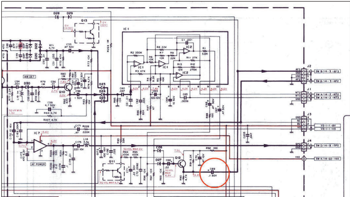
3 - Schéma de la partie de la carte "IF Unit" du TS-440, sur laquelle se trouve la chaîne BF. Quand on suit le cheminement des signaux BF, on passe successivement par : Q12, préampli ; C69, condensateur de couplage (qu'il va falloir enlever pour l'installation du module DSP) ; J2, connecteur du potentiomètre de volume ; IC7, ampli BF ; J4, connecteur du haut-parleur.
