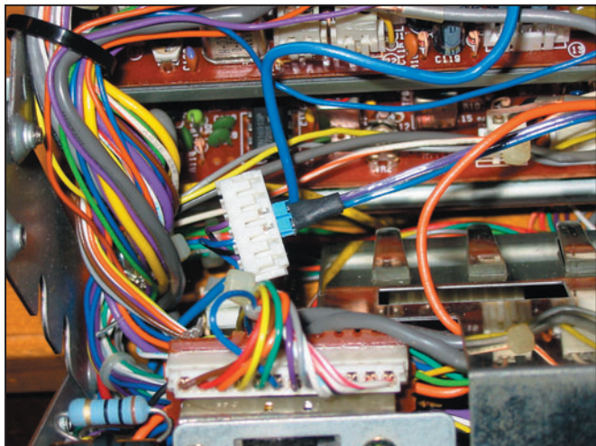
13 - Le câble de liaison qui a été réalisé est enfiché dans le connecteur J54 derrière la face avant. Ce connecteur n'est plus enfiché dans la carte "Control Unit" ; il n'est plus relié qu'au câble de liaison avec le module DSP.
