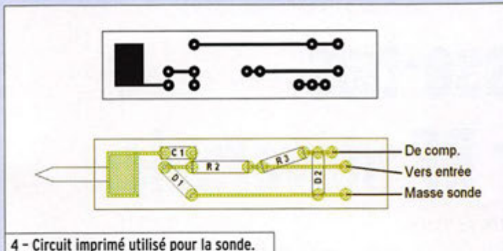
4 - Circuit imprimé utilisé pour la sonde.
