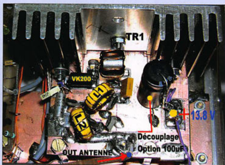
Photo 9 - Vue sur le PA. Les tores L1 et L2, détails.
