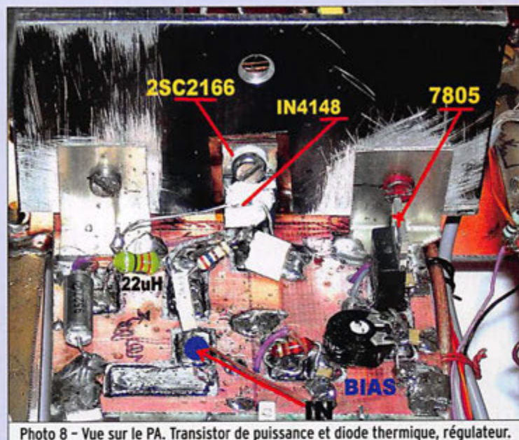
Photo 8 - Vue sur le PA. Transistor de puissance et diode thermique, régulateur.
