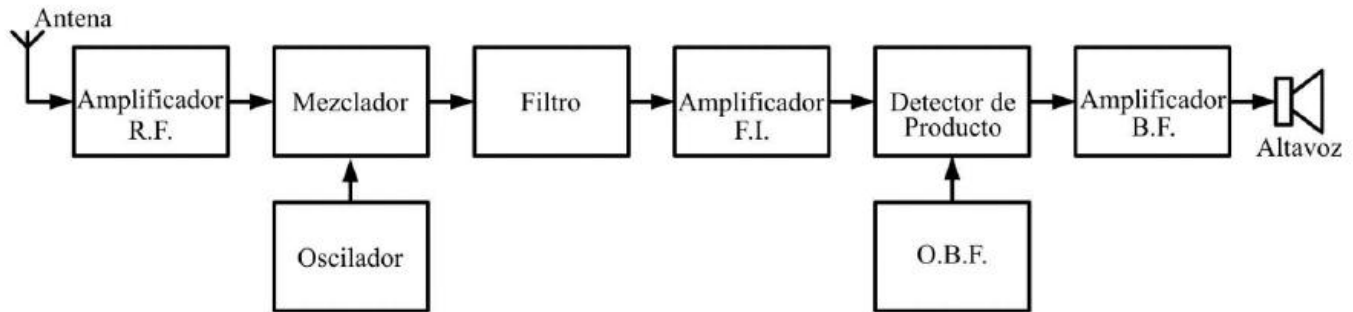
Receptor superheterodino de simple conversión
