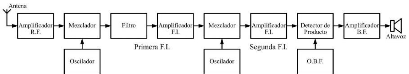
Receptor superheterodino de doble conversión
