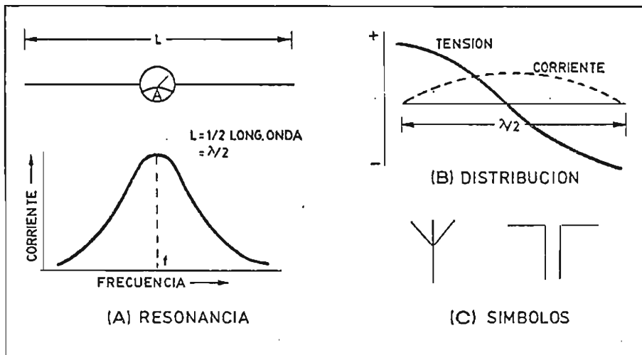
Fig. 58.R - Antena dipolo.
