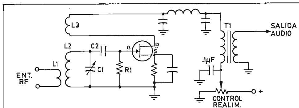
Fig. 54.R - Detector regenerativo (autodino).
