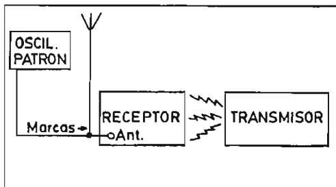
Fig. 70.R - Medida de frecuencia con marcador.
