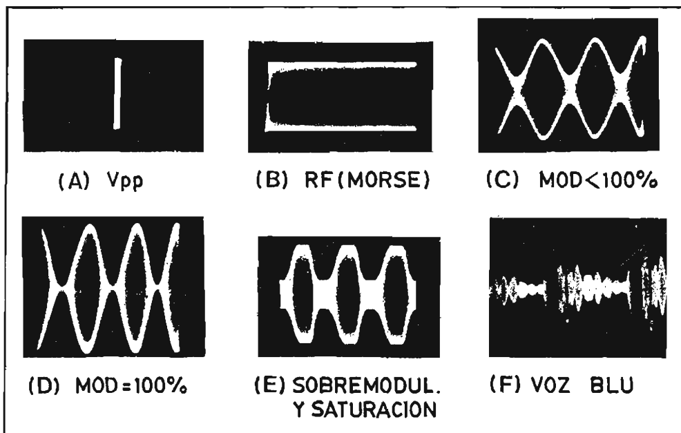
Fig. 74.R - Formas de onda en la pantalla osciloscópica.
