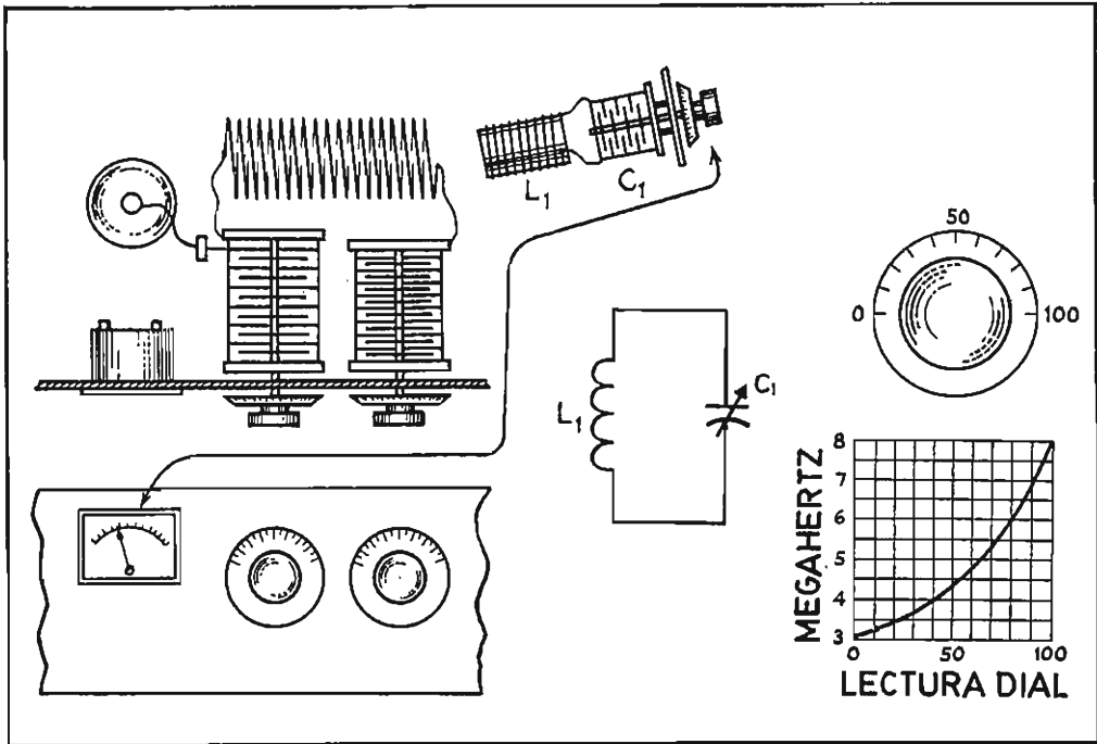
Fig. 71.R - Ondámetro de absorción para la medida de frecuencia.
