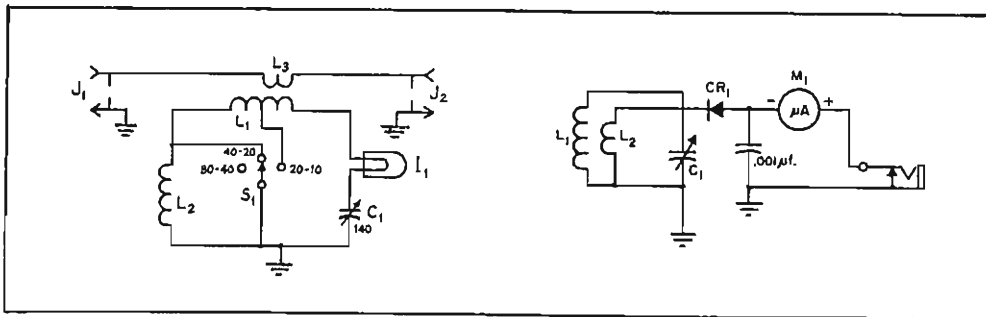
Fig. 72.R - Versiones prácticas del ondámetro de absorción.
