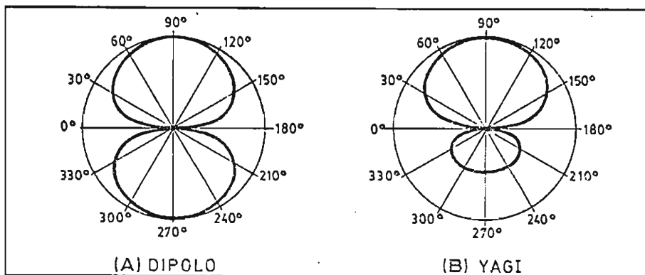
Fig. 60.R.- Directividad de la antena dipolo (A) y de la antena Yagi de tres elementos (B)
