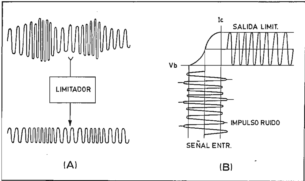
Fig. 51.R - Efecto (A) y proceso (B) del limitador.
