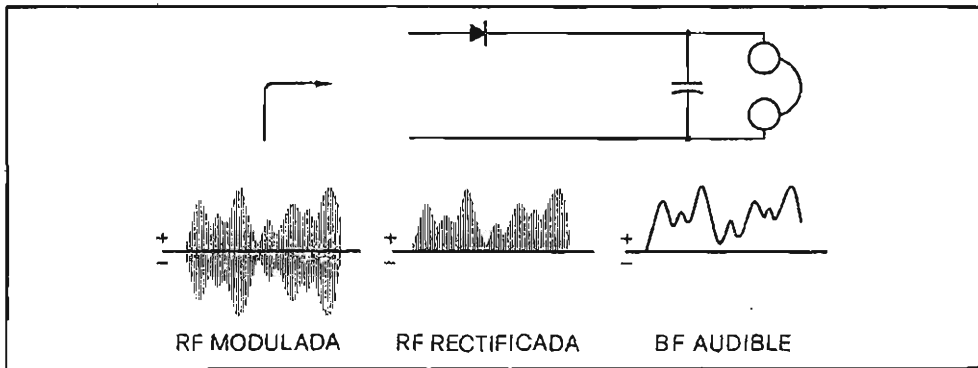
Fig. 46.R - Detector de AM.
