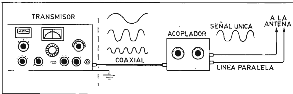
Fig. 67.R - Efecto filtro del acoplador de antena.
