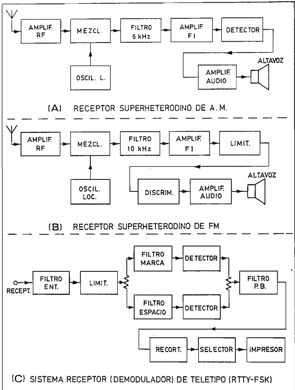
Fig. 56.R - Esquemas de bloques de
