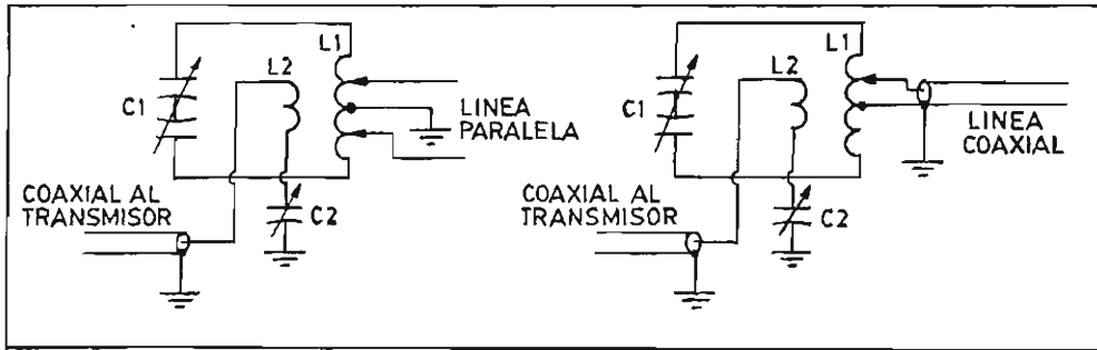
Fig. 66.R - Acopladores de antena.
