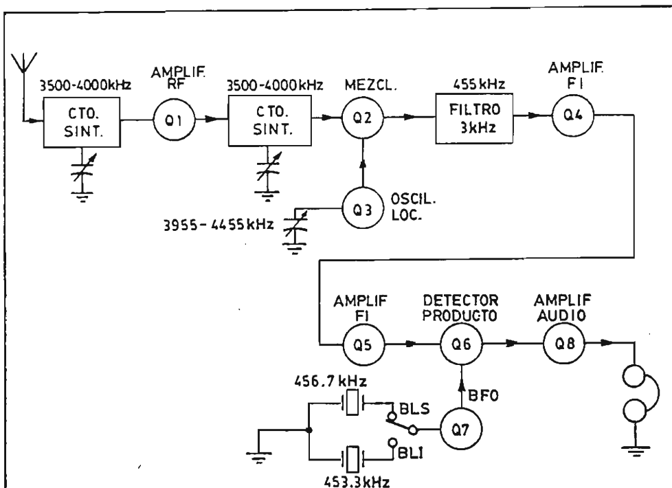
(D) MODERNO RECEPTOR DE BANDA LATERAL UNICA Y CW
