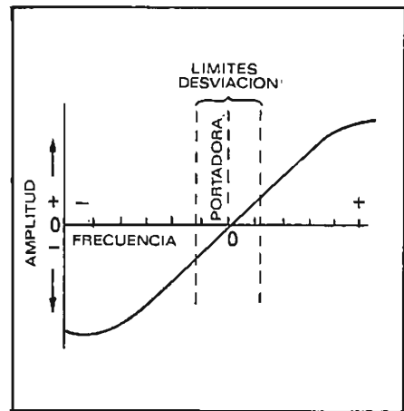
Fig. 52.R - Discriminador.
