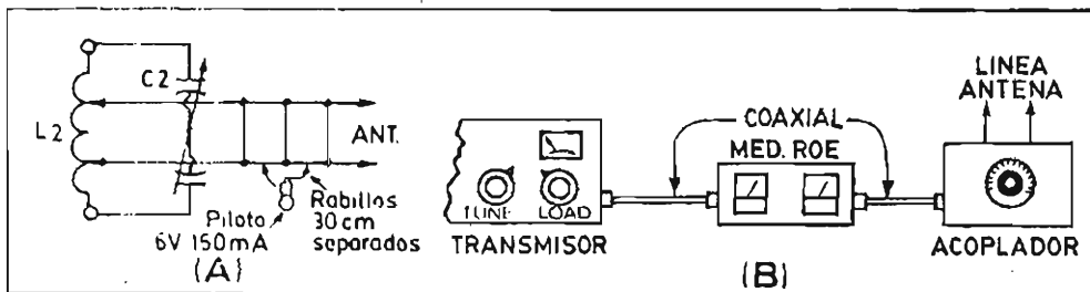
Fig. 73.R - Mediciones en el sistema de antena.
