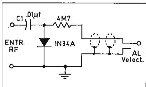
Fig. 69.R - Sonda de RF.
