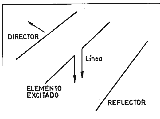
Fig. 62.R - Antena de gran directividad (Yagi).
