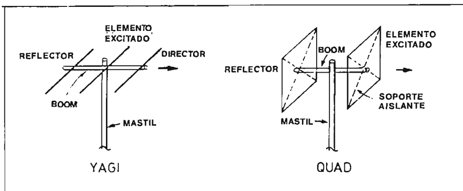
Fig. 63.R - Antenas directivas usuales
