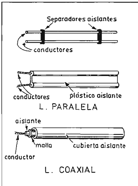
Fig. 65.R - Líneas de alimentación de antena.
