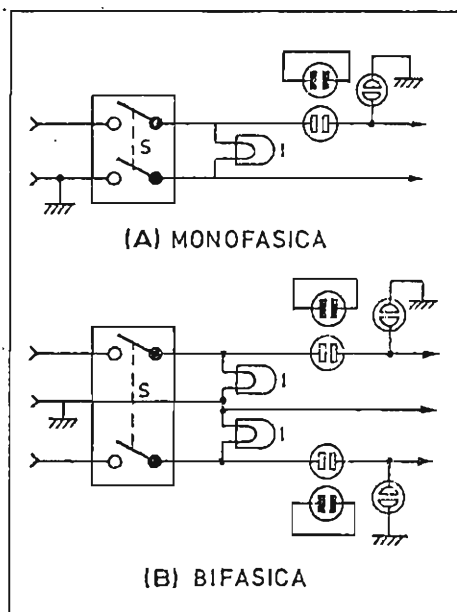
Fig. 78.R - Instalación general con protección.
