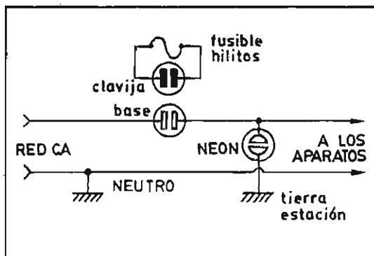
Fig. 77.R - Dispositivo de seguridad.
