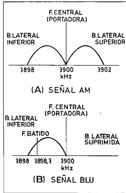
Fig. 49.R - Reinserción de portadora para detectar BLU.
