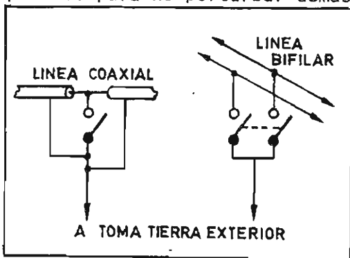
Fig. 68.R - Puesta a tierra de las antenas.
