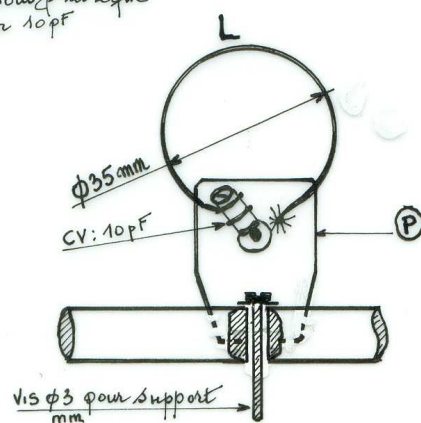
BOUCLE de COUPLAGE
