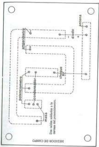
CARA "B": Visto el lado de componentes.
