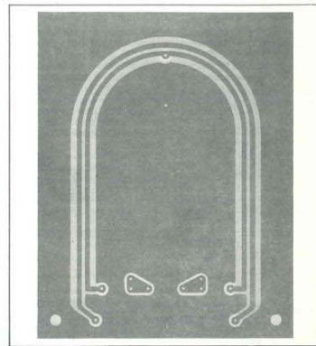
Figura 3.- Para frecuencias comprendidas entre 20 y 220 MHz, aconsejamos emplear este siguiente circuito, ya que es el más idóneo para VHF. Los valores de los componentes son idénticos para ambos circuitos, cosa que los valores indicados en el esquema eléctrico de la Figura 1.
