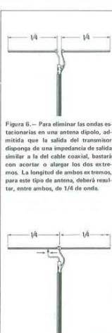
Figura 6.- Para eliminar las ondas estacionarias en una antena dipolo, admítase que la salida del transmisor disponga de una impedancia de salida similar a la del cable coaxial, bastará con acortar o alargar los dos extremos. La longitud de ambos extremos, para este tipo de antena, deberá resultar, entre otros, de 1/4 de onda.
